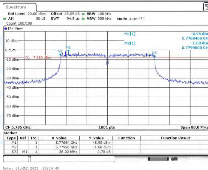
11AC40MIMO_Ant4_5795
