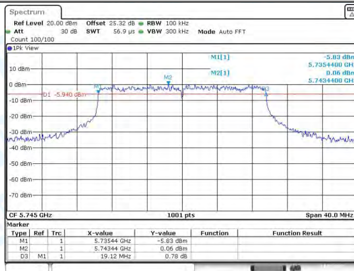
11AX20MIMO_Ant4_5745
