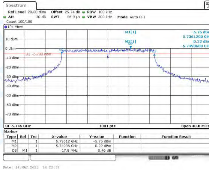
11AC20MIMO_Ant3_5745
