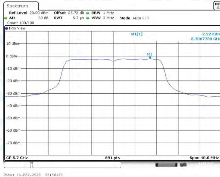
11N20MIMO_Ant3_5700
