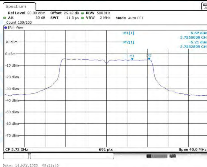
11N20MIMO_Ant4_5720_UNII-3
