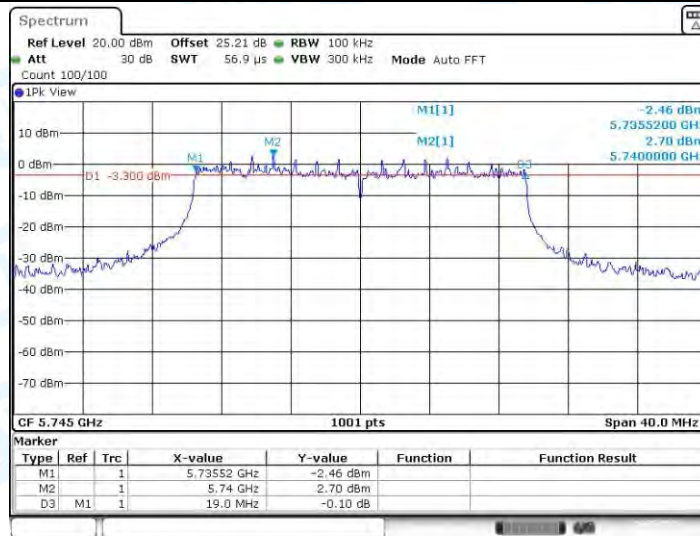
11AX20MIMO_Ant3_5745
