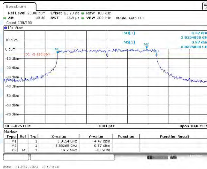
11AX20MIMO_Ant3_5825
