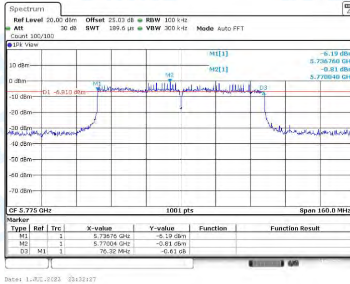
11AC80MIMO_Ant4_5775
