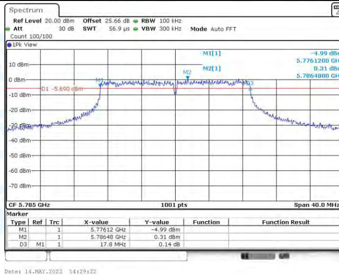
11AC20MIMO_Ant3_5785
