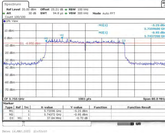
11AX40MIMO_Ant4_5755
