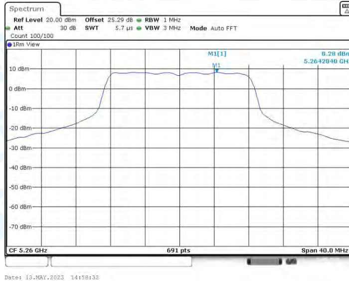
11A_Ant3_5260
