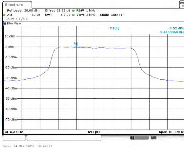
11N20MIMO_Ant4_5500
