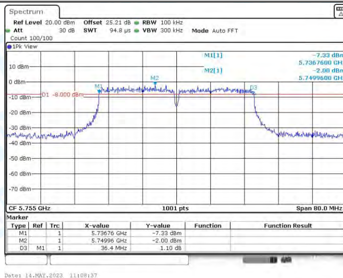
11N40MIMO_Ant4_5755
