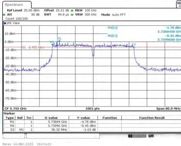
11AC40MIMO_Ant4_5755
