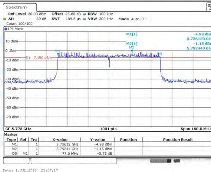
11AX80MIMO_Ant3_5775
