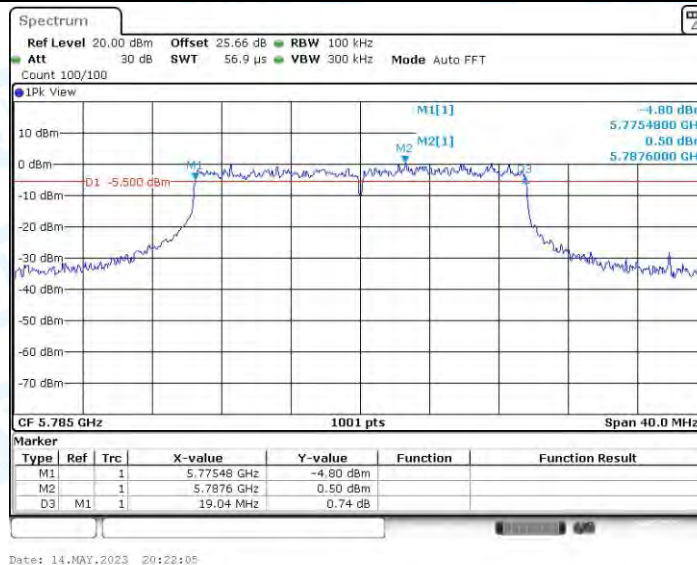
11AX20MIMO_Ant3_5785
