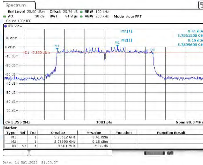
11AX40MIMO_Ant3_5755
