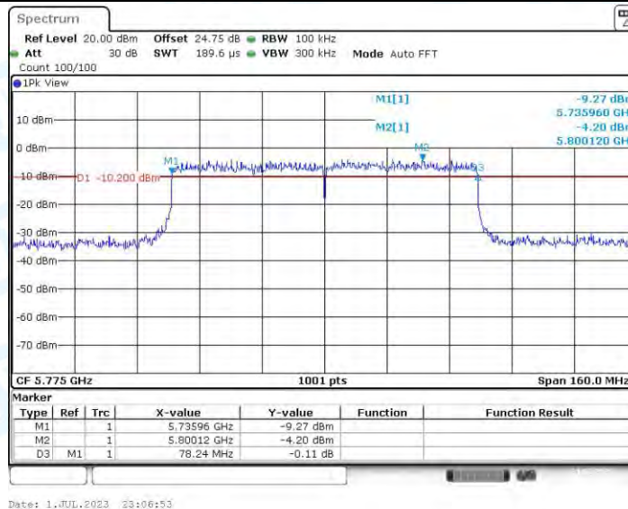
11AX80MIMO_Ant2_5775
