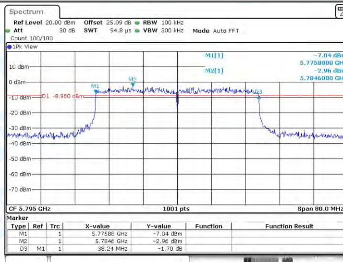
11AX40MIMO_Ant3_5795
