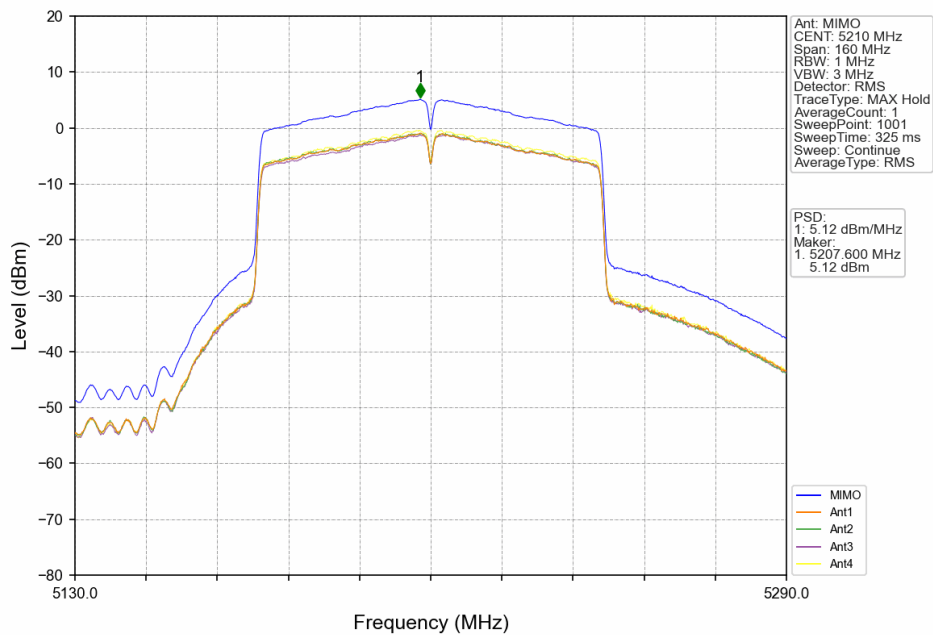
802.11ac(VHT80)_MCH_5210MHz_MIMO_NTNV
