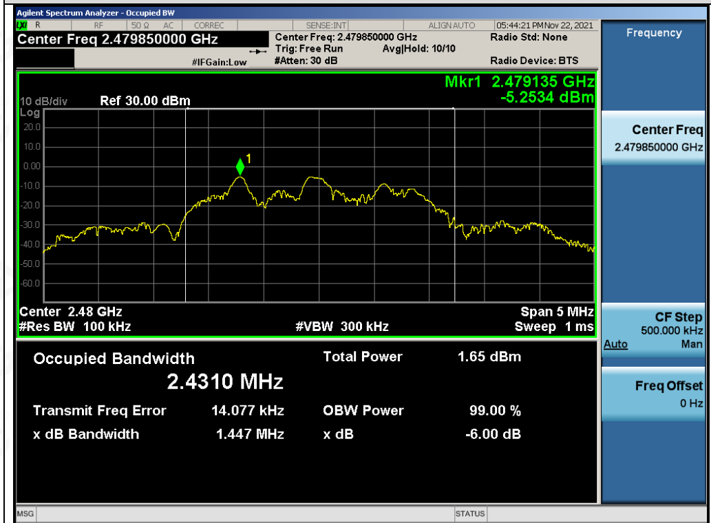
Test_Graph_ANT1_2479.85_DTSBW
