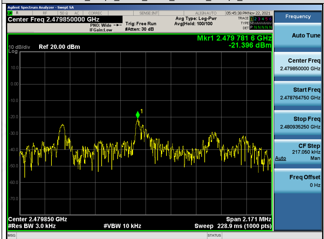
Test_Graph_LE2M_ANT1_2479.85_2Mbps_PSD
