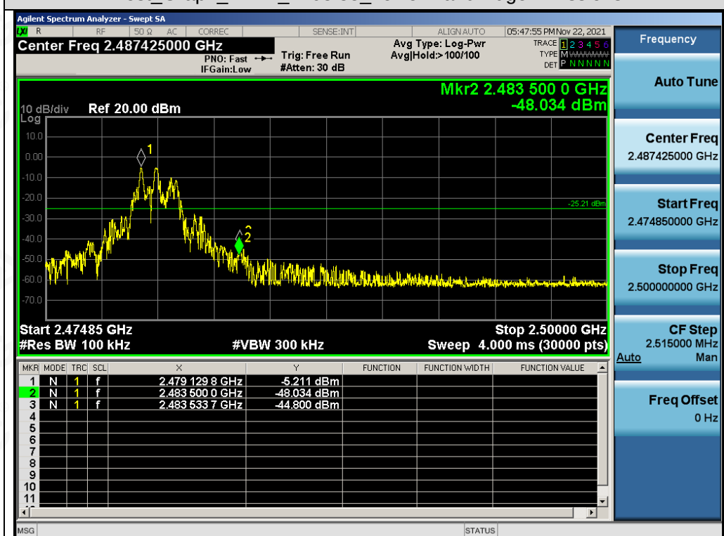
Test_Graph_ANT1_2479.85_Higher Band Edge Emissions
