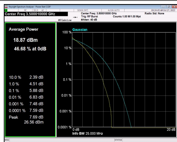
n77(3450-3550) SCS=30kHz DFT_QPSK BW=20MHz Channel=633334 RB=50@0
