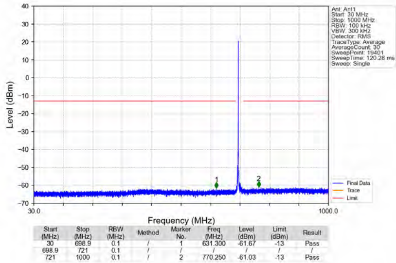
n12_15kHz_SISO_NTNV_10MHz_DFT-s-OFDM_PI/2_BPSK_707.5MHz_Edge_1RB_Left
