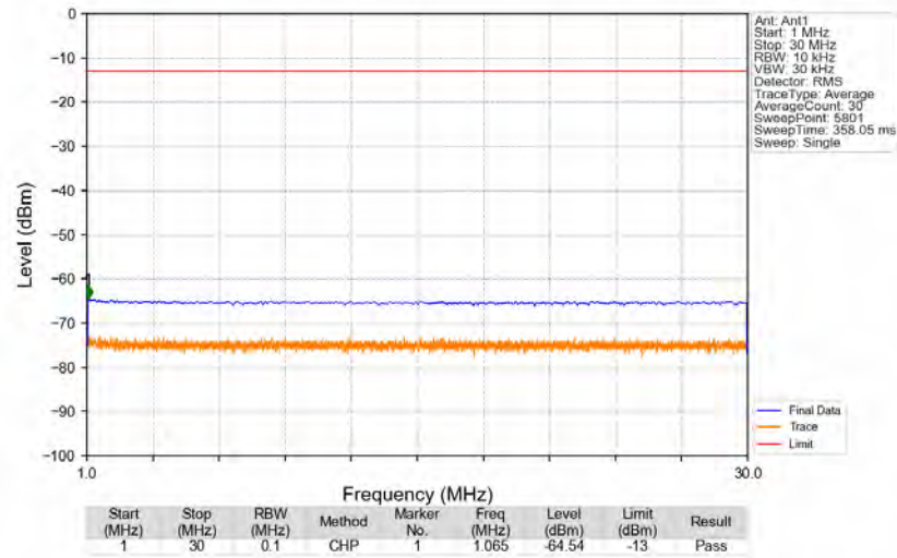
n12_15kHz_SISO_NTNV_10MHz_DFT-s-OFDM_PI/2_BPSK_707.5MHz_Edge_1RB_Left
