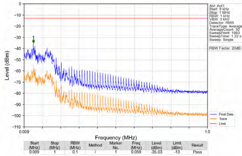
n12_15kHz_SISO_NTNV_10MHz_DFT-s-OFDM_PI/2_BPSK_707.5MHz_Edge_1RB_Left
