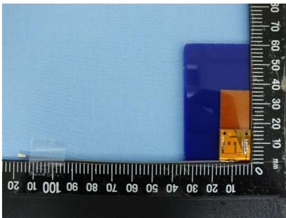
ANT.: PIFA, P/N: EFB2471A3S-10MH4L
