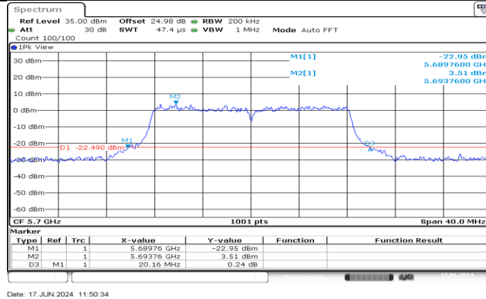
11A-CDD_Ant1_5700
