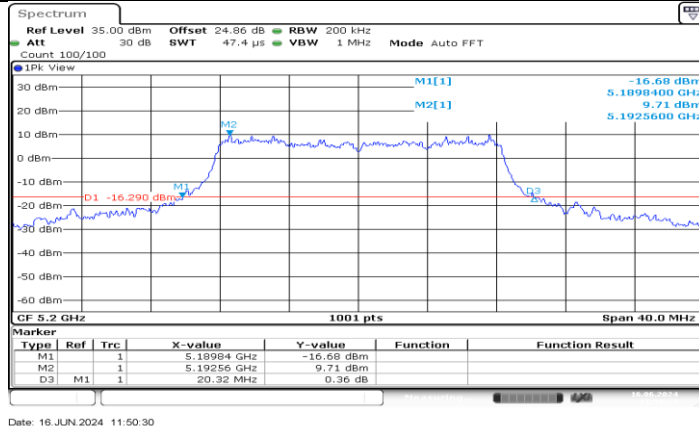
11A-CDD_Ant3_5200
