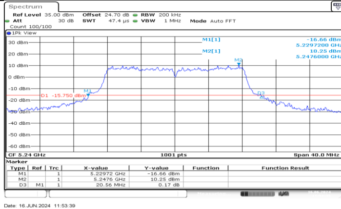
11A-CDD_Ant1_5240
