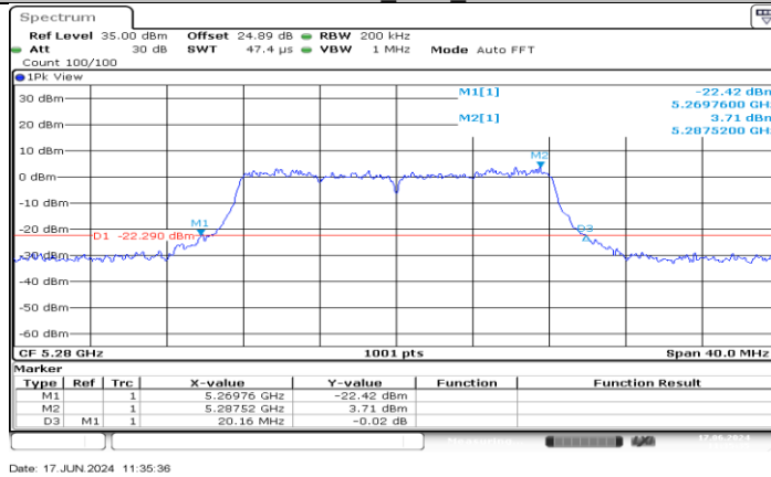
11A-CDD_Ant1_5280
