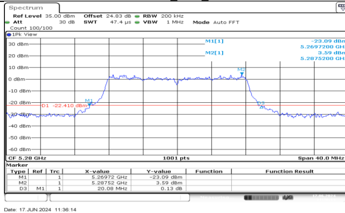
11A-CDD_Ant2_5280
