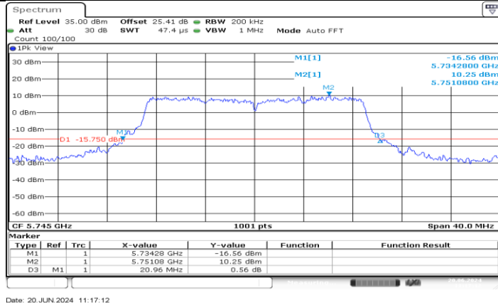
11AC20MIMO_Ant3_5745
