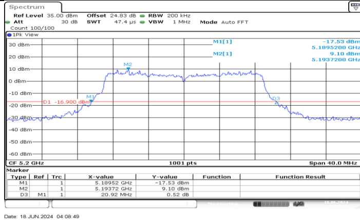
11AC20MIMO_Ant2_5200
