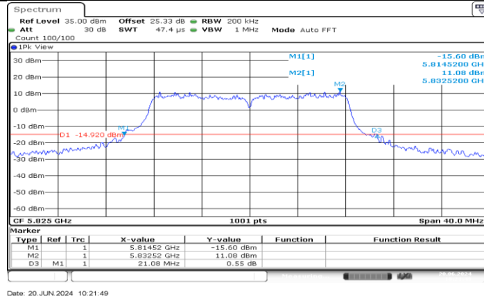
11A-CDD_Ant1_5825
