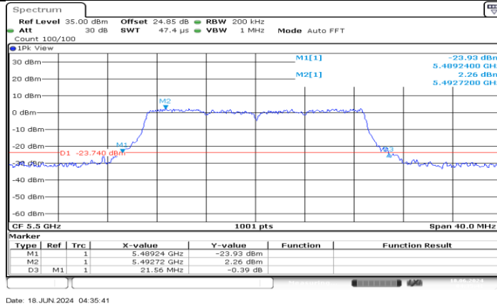
11AC20MIMO_Ant2_5500
