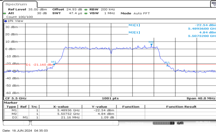
11AC20MIMO_Ant1_5500
