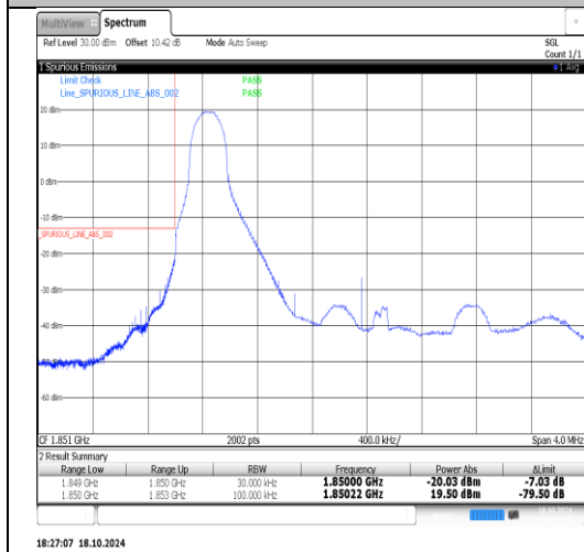
Band2-3MHz-QPSK-18615-1RB#14-PASS
