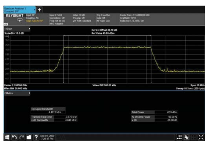
Figure 373: QPSK 5MHz B.W; 2155MHz – 4G OUTPUT
