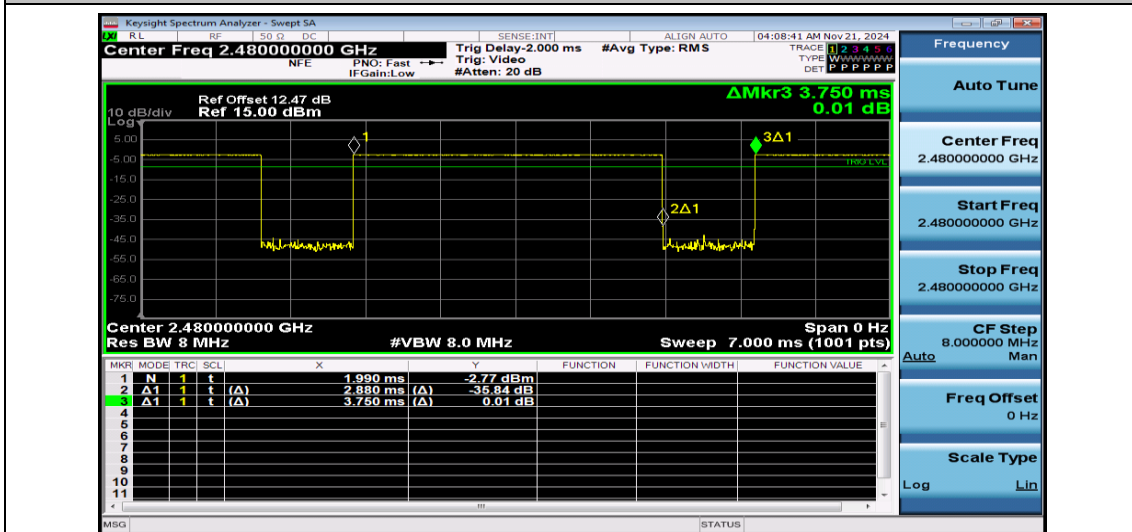
NTNV-DH5-Ant1-2480
