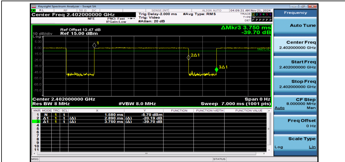
NTNV-2DH5-Ant1-2402
