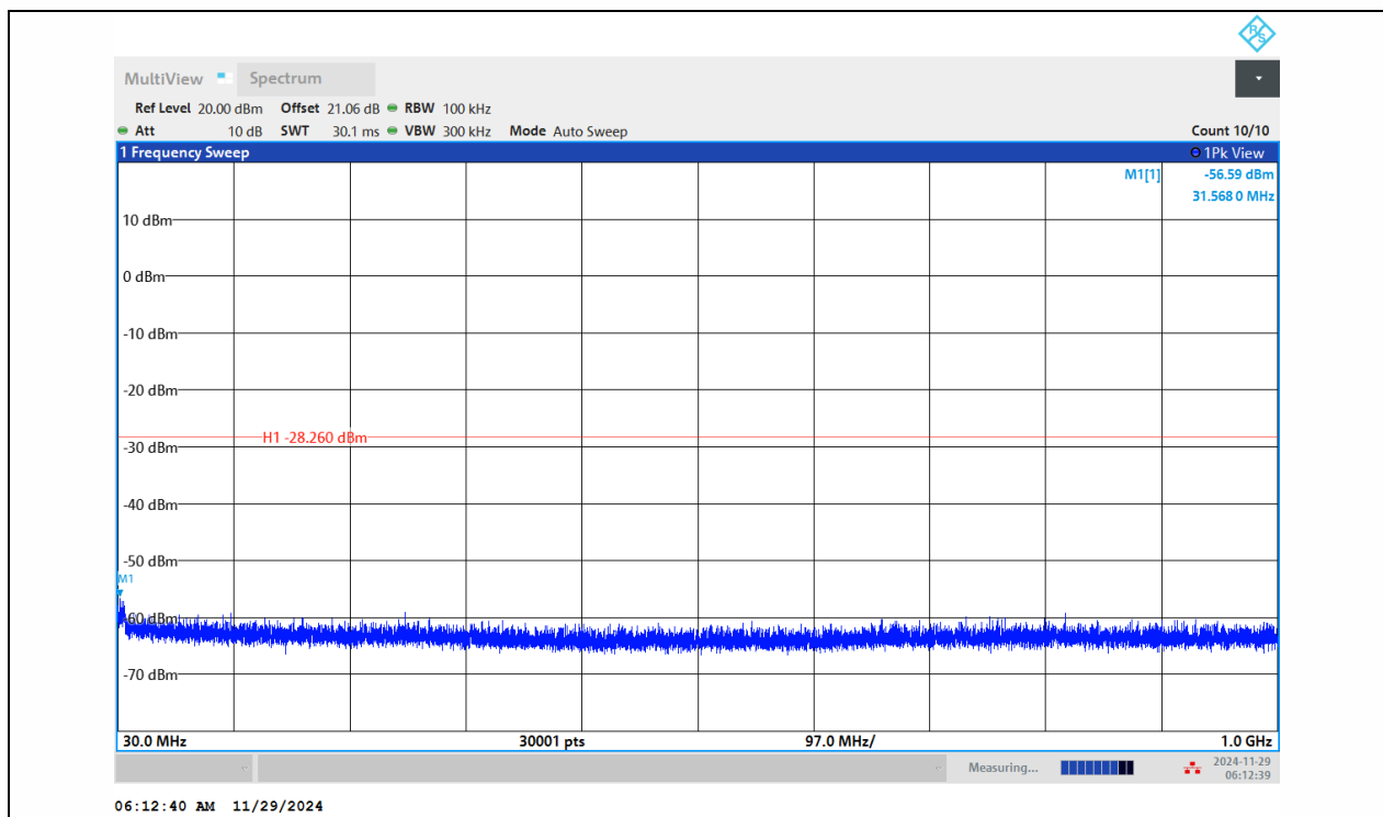
11G-Ant1-2437-30~1000-PASS
