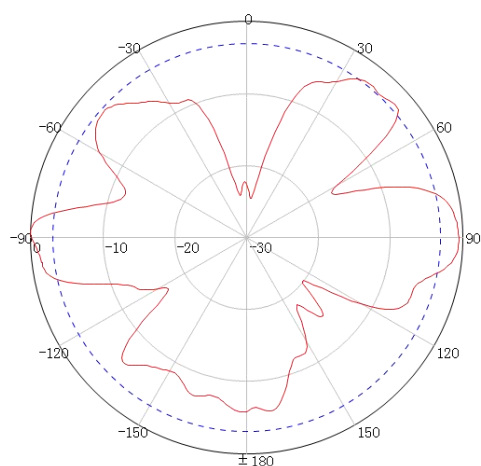
E 面 (4900MHz)
