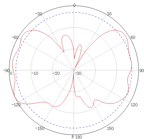
E 面 (1470MHz)
