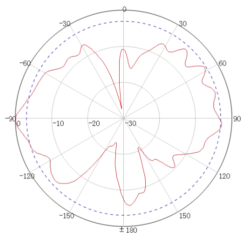
E 面 (5900MHz)
