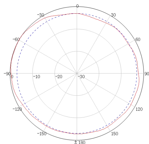
H 面 (5550MHz)
