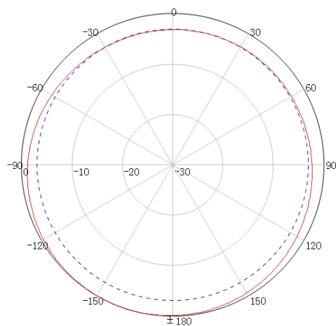
H 面 (1470MHz)
