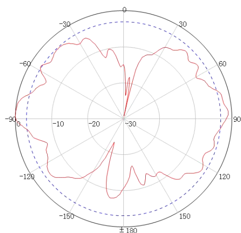
E 面 (5550MHz)
