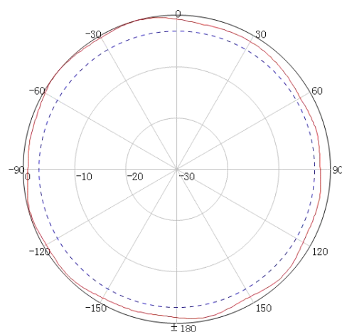
H 面 (4900MHz)
