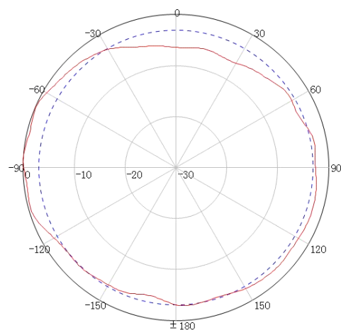
H 面 (5900MHz)
