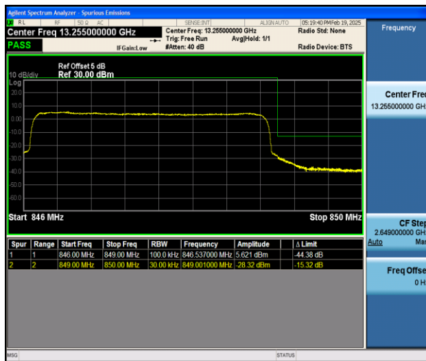
Band5_3MHz_QPSK_20635_15RB#0
