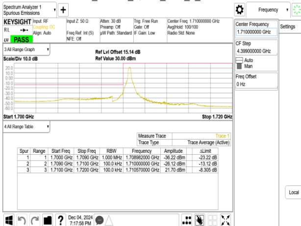
Band4_10MHz_QPSK_RB50_0_CH20000
