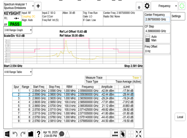
Band7_5MHz_QPSK_RB1_24_CH21425
