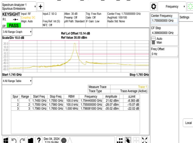
Band4_10MHz_QPSK_RB1_49_CH20350
