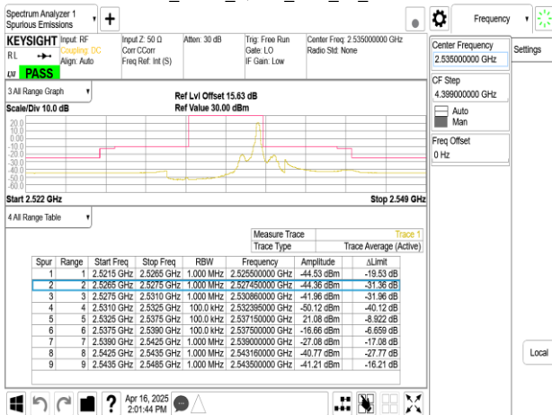
Band7_5MHz_QPSK_RB1_24_CH21100
