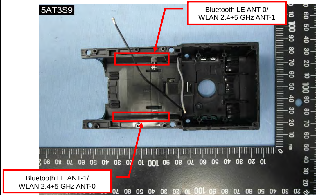
EUT Photo (64)
