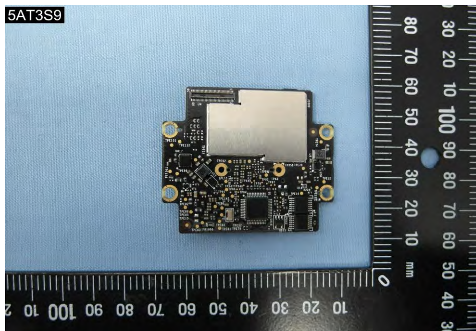
EUT Photo (48)
