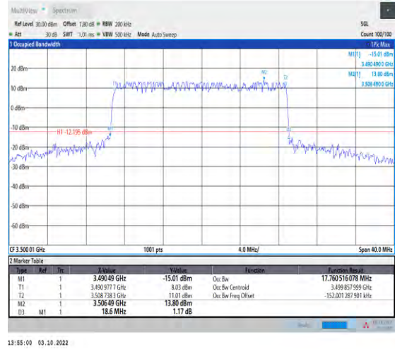
1-N78-3450-3550--30-20-M-1-DFT-QPSK-Outer_Full -50@0-Ant1-17.761-18.600-≤20-PASS
