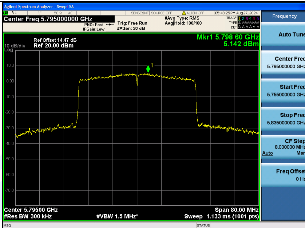
11AX40MIMO-Ant3-5795-PASS
