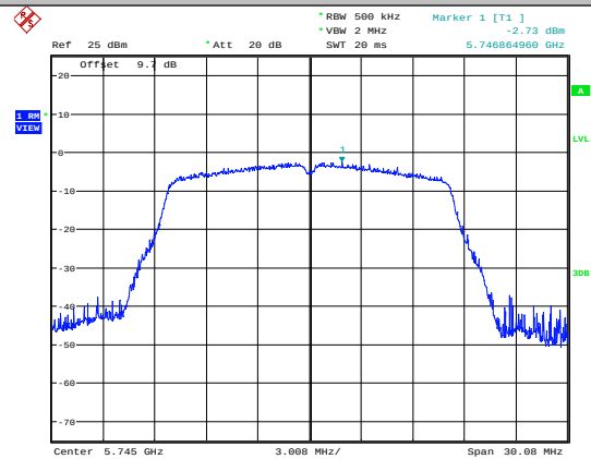
11A-Ant1-5745
