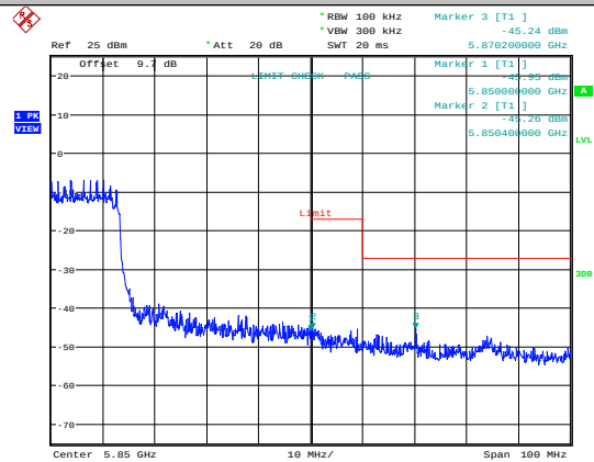
11AC80SISO-Ant1-5775
