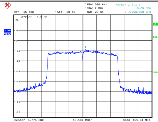
11AC80SISO-Ant1-5775
