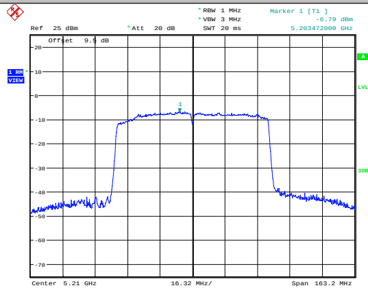
11AC80SISO-Ant1-5210
