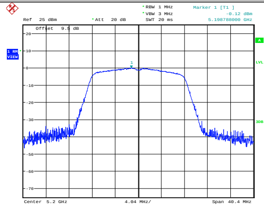
11A-Ant1-5200
