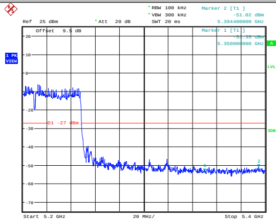
11AC80SISO-Ant1-5210
