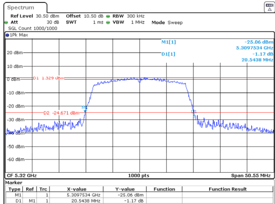
802.11ac20_5320MHz
