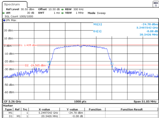
802.11ac20_5260MHz
