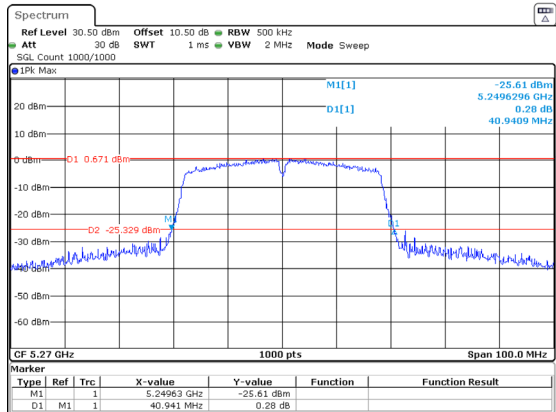
802.11ac40_5270MHz
