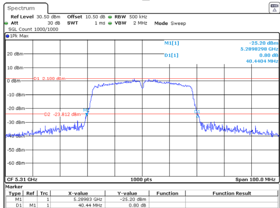
802.11ac40_5310MHz
