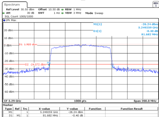
802.11ac80_5290MHz
