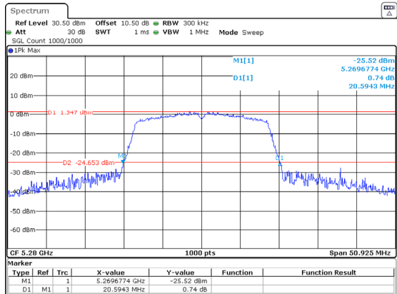
802.11ac20_5280MHz
