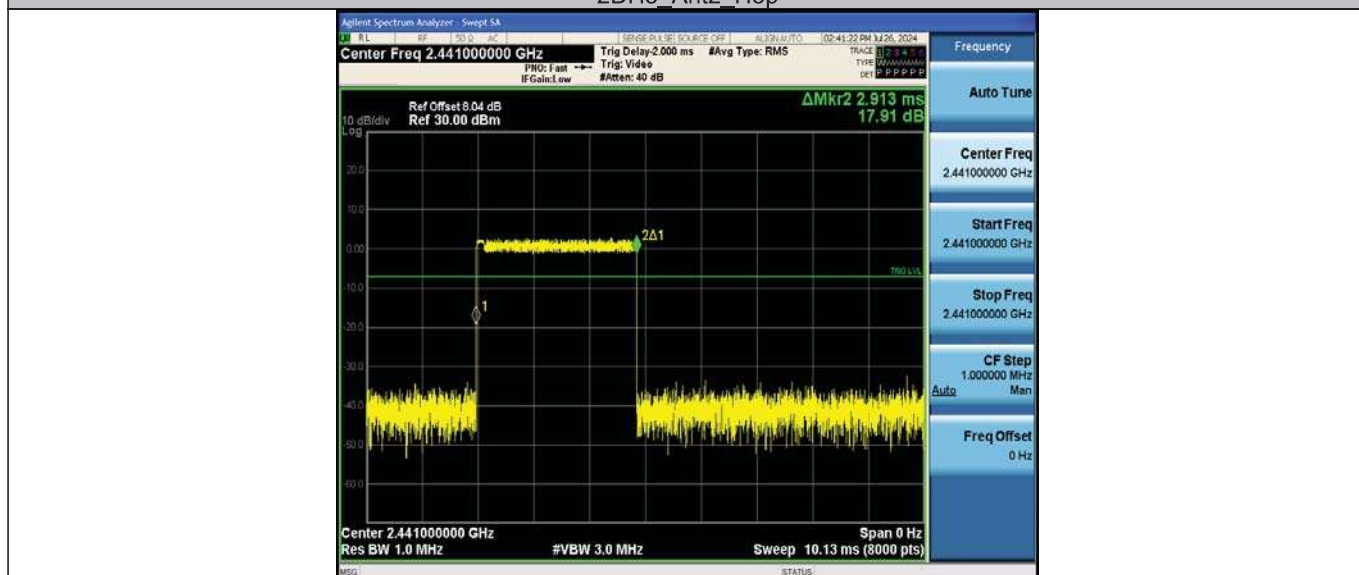
2DH5_Ant2_Hop
