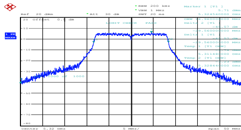
a_5320MHz_Chain 0
