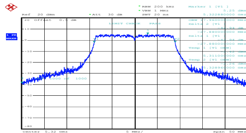
n20_5320MHz_Chain 0
