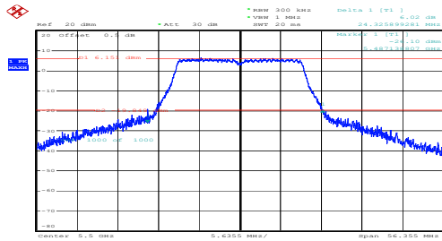
n20_5500MHz_Chain 0
