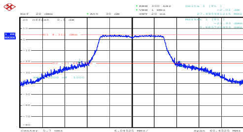
n20_5700MHz_Chain 0
