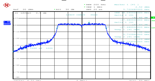
n20_5720MHz_Chain 0
