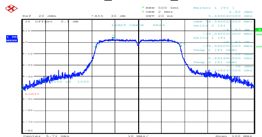
n40_5710MHz_Chain 0
