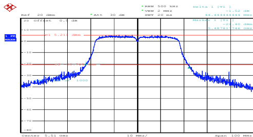
n40_5510MHz_Chain 0
