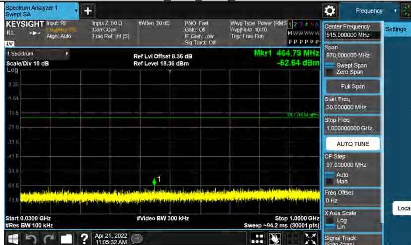
DH5 Ant1 2402 30~1000
