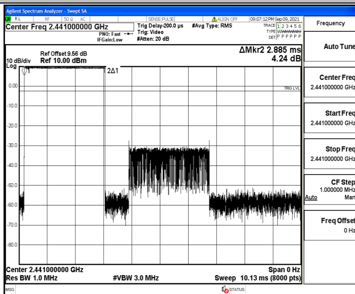
DH5_Ant3_Hop
