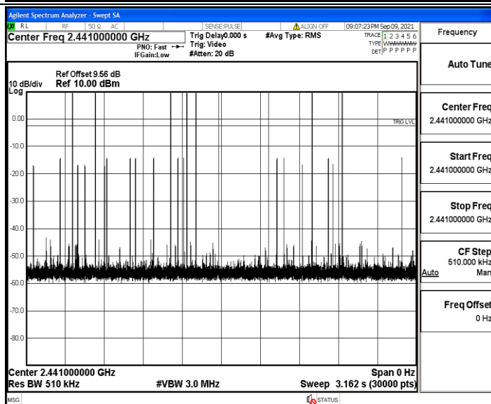
2DH5_Ant3_Hop
