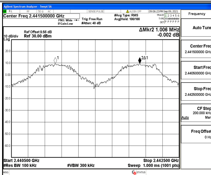
2DH5_Ant3_Hop
