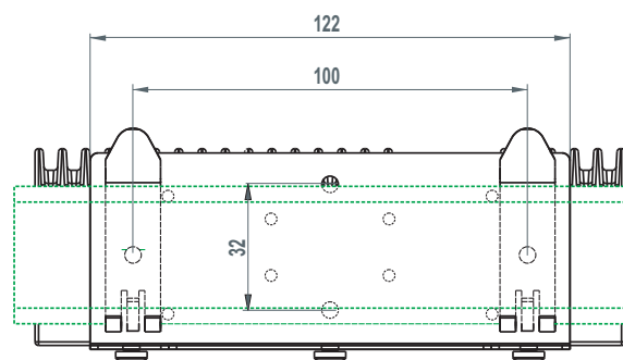
Fig. 4.21: L-bracket
