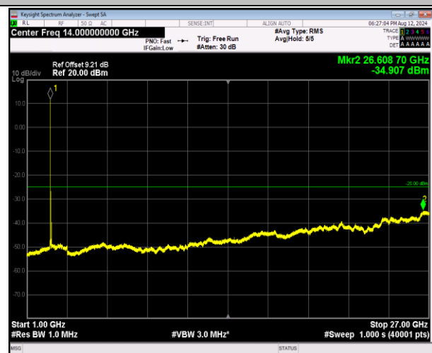
7-7-20MHz-20MHz-QPSK-QPSK-21001-21199-1RB#0-1 RB#99-1000~27000MHz-PASS
