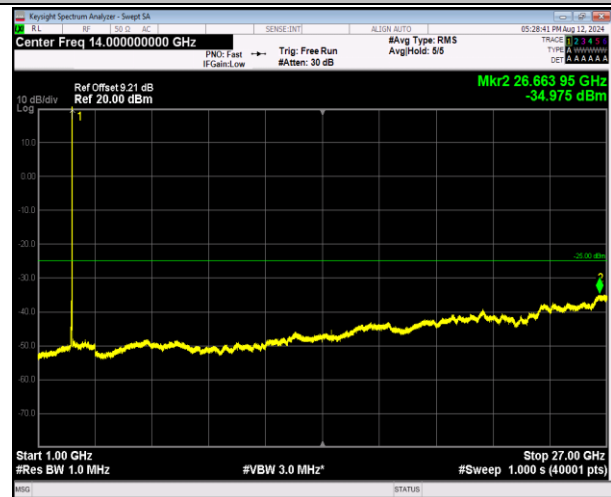
7-7-20MHz-10MHz-QPSK-QPSK-21251-21395-1RB#99-0 RB#0-1000~27000MHz-PASS
