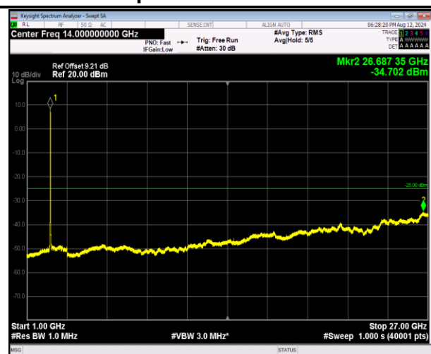
7-7-20MHz-20MHz-QPSK-QPSK-21001-21199-100RB#0- 100RB#0-1000~27000MHz-PASS
