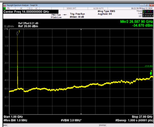
7-7-20MHz-20MHz-QPSK-QPSK-20850-21048-1RB#0-1 RB#99-1000~27000MHz-PASS
