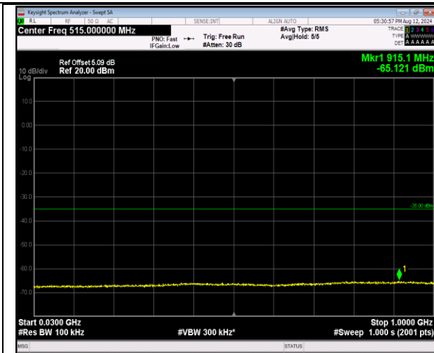
7-7-20MHz-10MHz-QPSK-QPSK-21251-21395-100RB# 0-50RB#0-30~1000MHz-PASS
