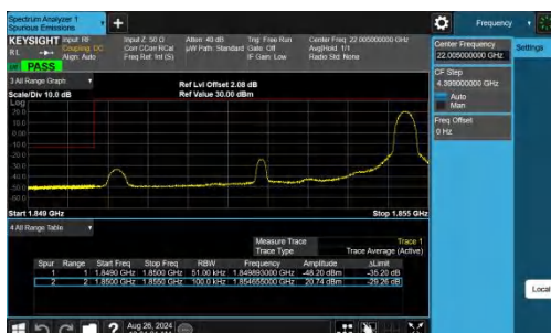
Band2-5MHz-QPSK-18625-1RB#24-PASS
