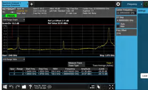
Band2-20MHz-QPSK-18700-1RB#99-PASS
