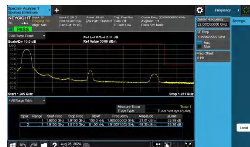
Band2-5MHz-QPSK-19175-1RB#0-PASS
