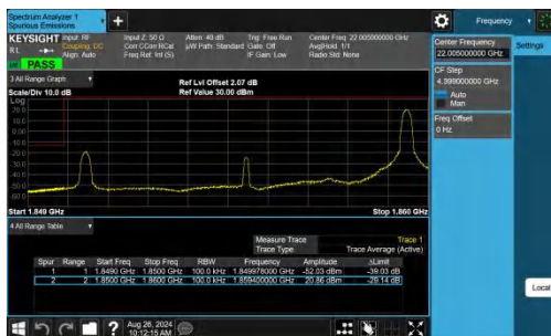
Band2-10MHz-QPSK-18650-1RB#49-PASS
