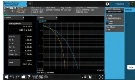
Band2-20MHz-16QAM-18900-27RB#0-PASS
