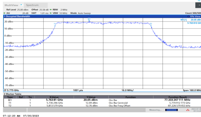
11AC80MIMO_Ant2_5775
