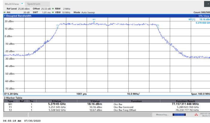
11AC80MIMO_Ant2_5290
