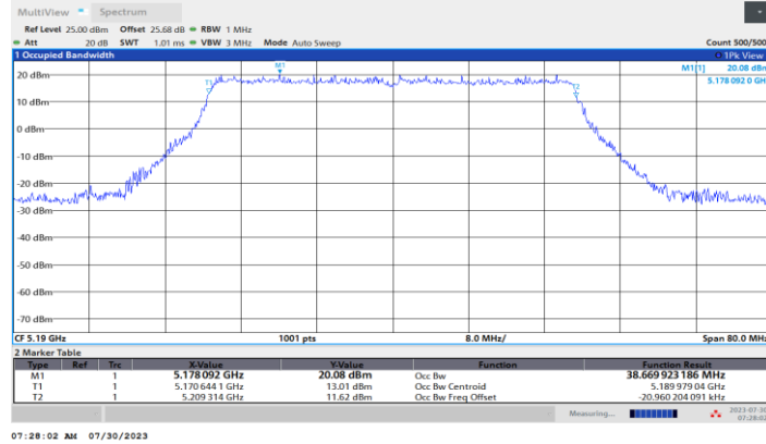
11BE40MIMO_Ant1_5190
