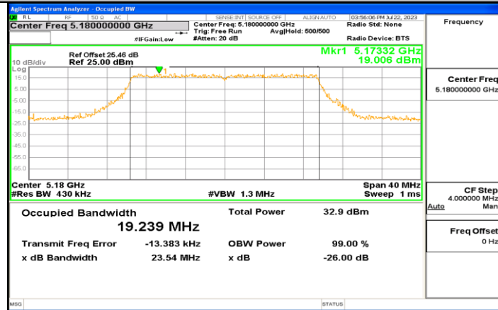
11BE20MIMO_Ant1_5180
