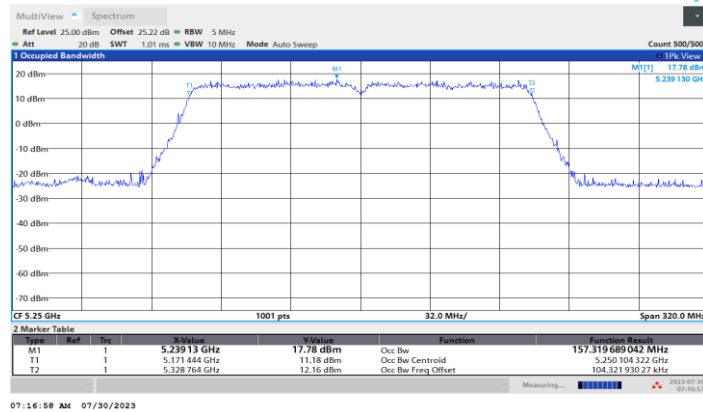
11AC160MIMO_Ant2_5250
