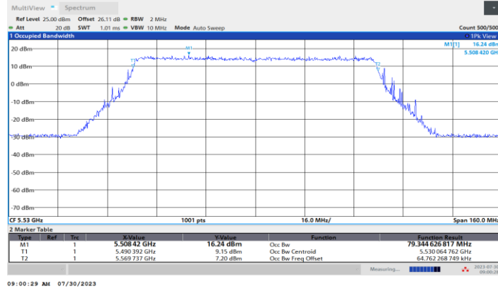
11BE80MIMO_Ant1_5530
