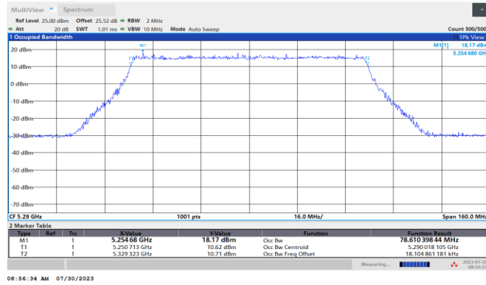
11BE80MIMO_Ant1_5290
