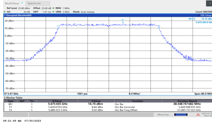
11BE40MIMO_Ant1_5670
