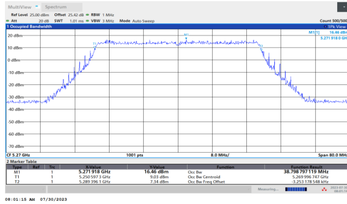
11BE40MIMO_Ant1_5270
