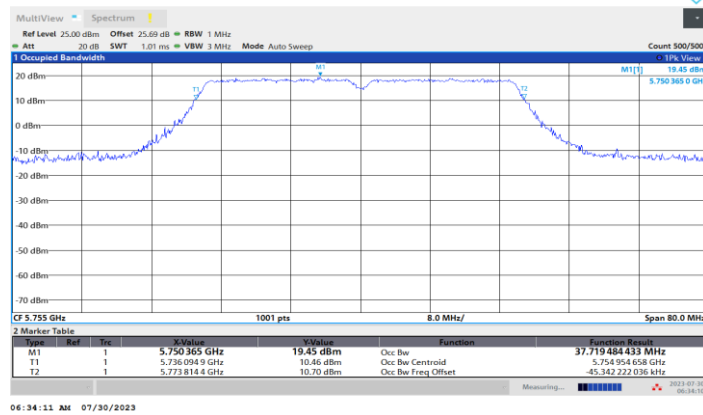
11AC40MIMO_Ant1_5755
