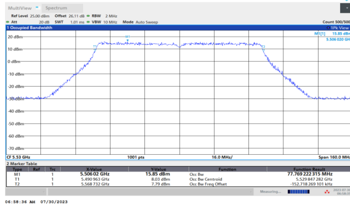
11AC80MIMO_Ant1_5530
