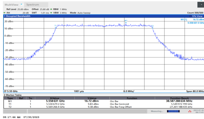
11BE40MIMO_Ant1_5550
