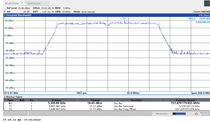
11AC160MIMO_Ant2_5570
