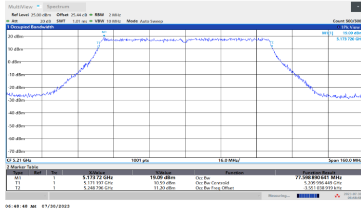
11AC80MIMO_Ant1_5210
