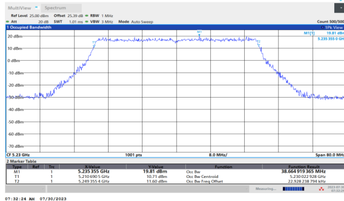
11BE40MIMO_Ant1_5230
