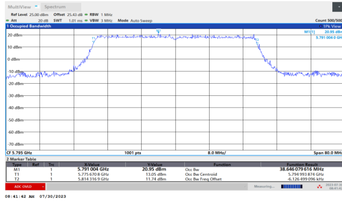
11BE40MIMO_Ant2_5795
