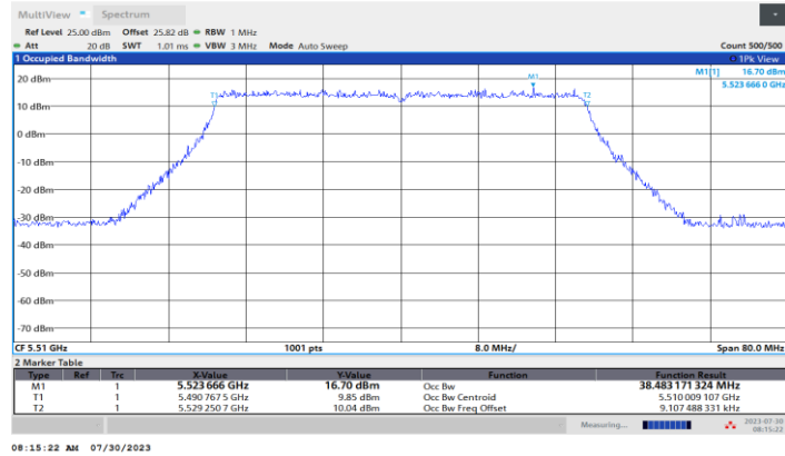
11BE40MIMO_Ant2_5510
