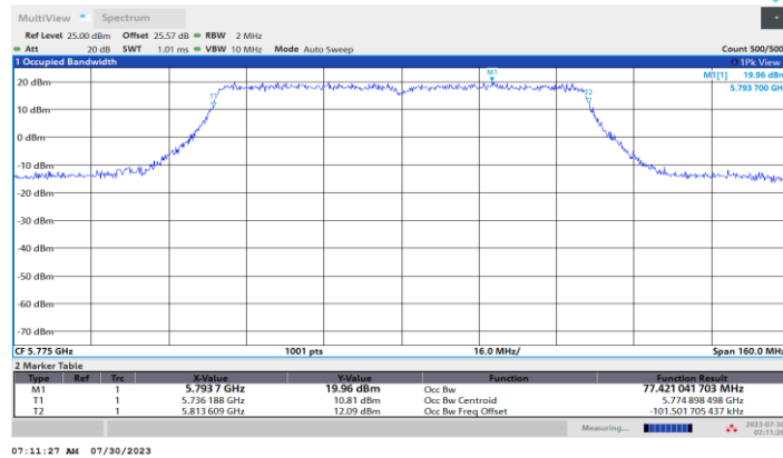
11AC80MIMO_Ant1_5775
