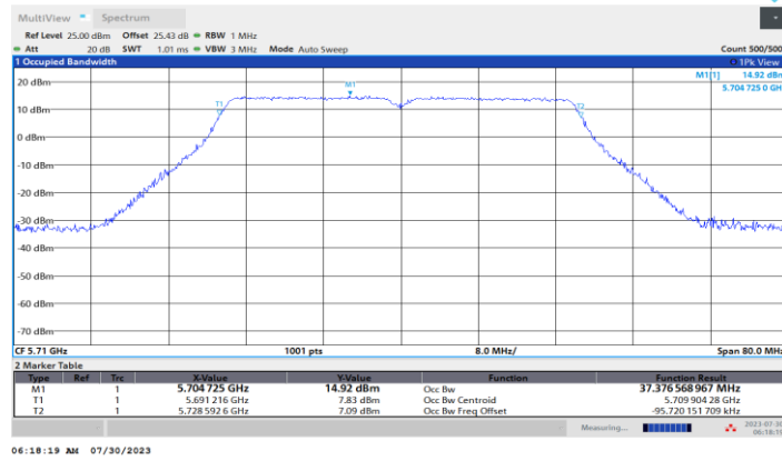
11AC40MIMO_Ant2_5710
