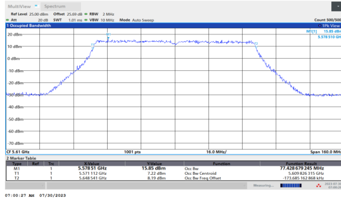
11AC80MIMO_Ant1_5610
