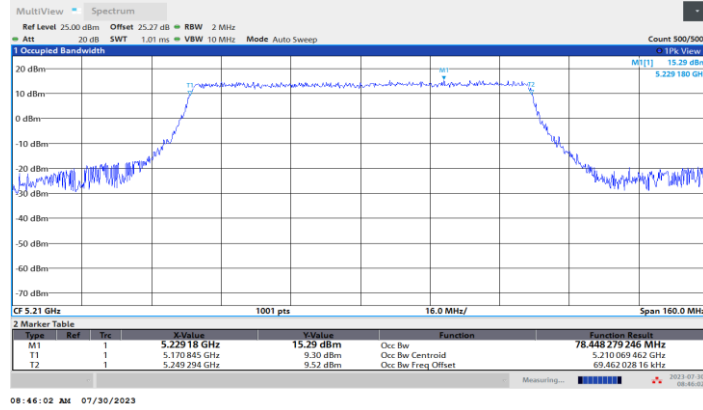
11BE80MIMO_Ant2_5210
