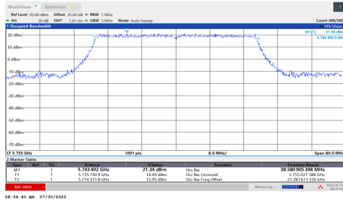
11BE40MIMO_Ant1_5755
