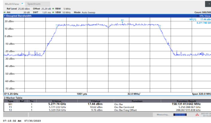
11AC160MIMO_Ant1_5250
