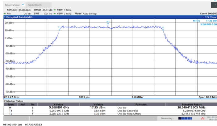
11BE40MIMO_Ant2_5270
