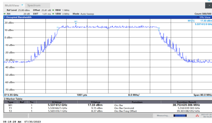
11BE40MIMO_Ant2_5550
