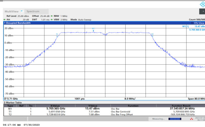
11AC40MIMO_Ant1_5710
