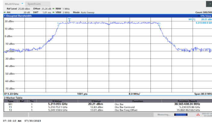
11BE40MIMO_Ant2_5230
