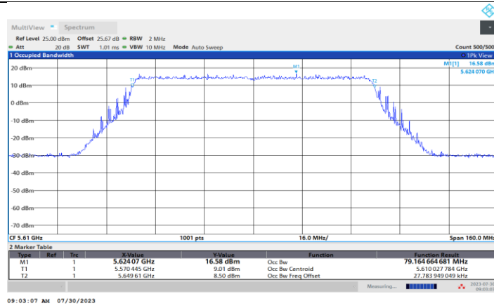
11BE80MIMO_Ant2_5610
