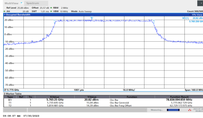
11BE80MIMO_Ant1_5775
