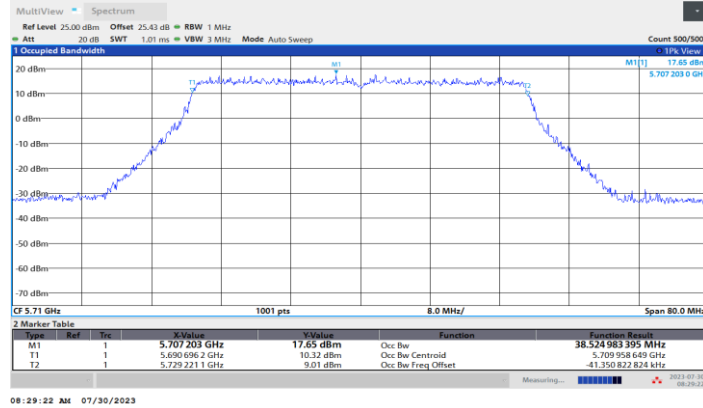
11BE40MIMO_Ant2_5710
