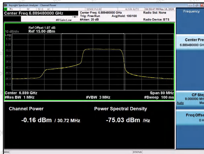
11AX40SISO-Ant1-6885-242Tone-RU62-PASS
