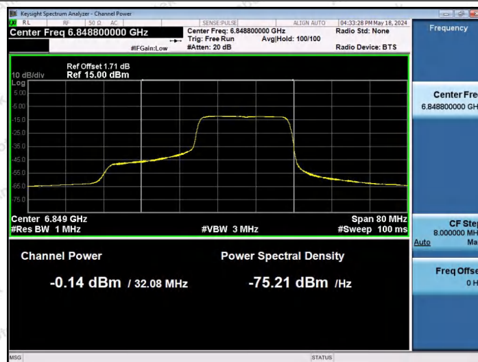
11AX40SISO-Ant1-6845-242Tone-RU62-PASS
