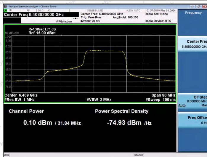
11AX40SISO-Ant1-6405-242Tone-RU62-PASS
