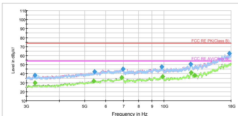
RE 3-18GHz PK+AV
