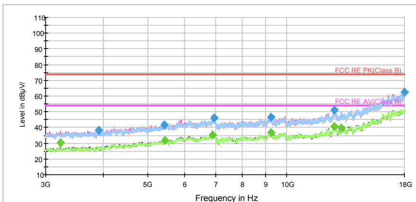
RE 3-18GHz PK+AV
