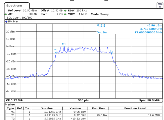
802.11ac20_5720MHz_Chain 1
