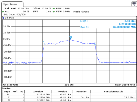
802.11ac80_5290MHz_Chain 2
