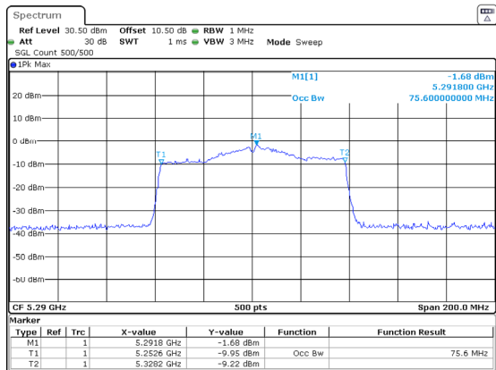
802.11ac80_5290MHz_Chain 1
