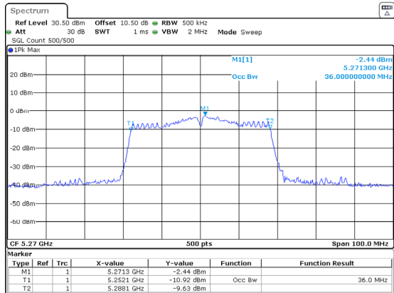
802.11ac40_5270MHz_Chain 1
