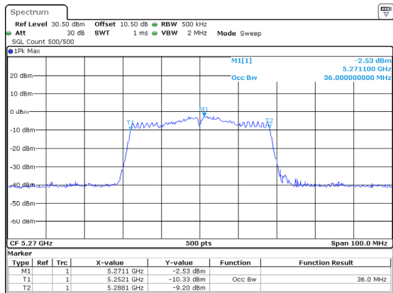
802.11ac40_5270MHz_Chain 2
