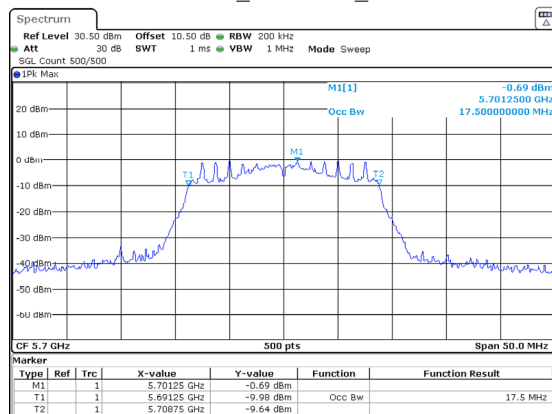
802.11ac20_5700MHz_Chain 1
