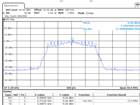
802.11ac20_5280MHz_Chain 2
