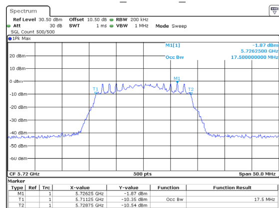
802.11ac20_5720MHz_Chain 2
