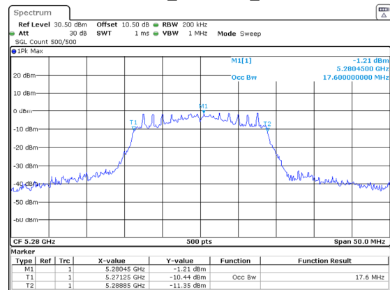
802.11ac20_5280MHz_Chain 1
