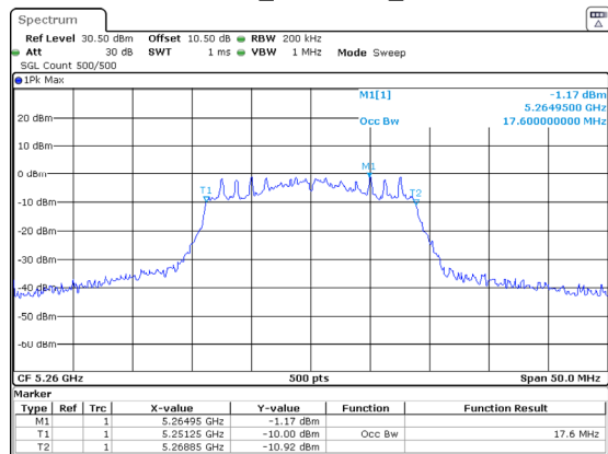
802.11ac20_5260MHz_Chain 1
