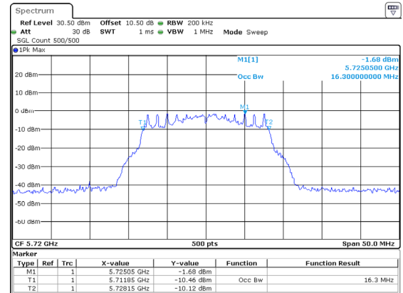
802.11a_5720MHz_Chain 2
