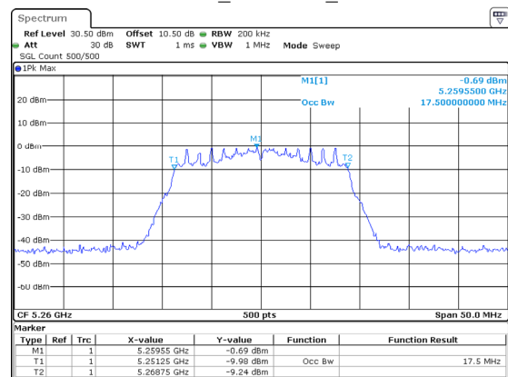
802.11ac20_5260MHz_Chain 2
