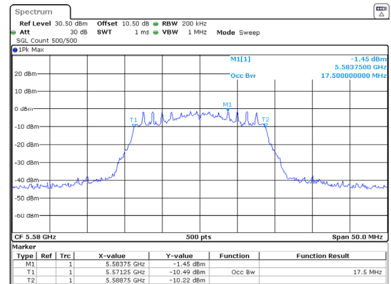
802.11ac20_5580MHz_Chain 1
