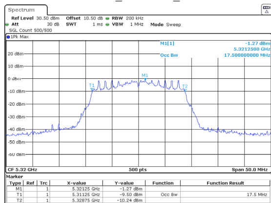
802.11ac20_5320MHz_Chain 1
