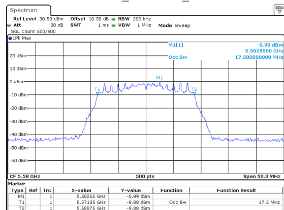
802.11ac20_5580MHz_Chain 2
