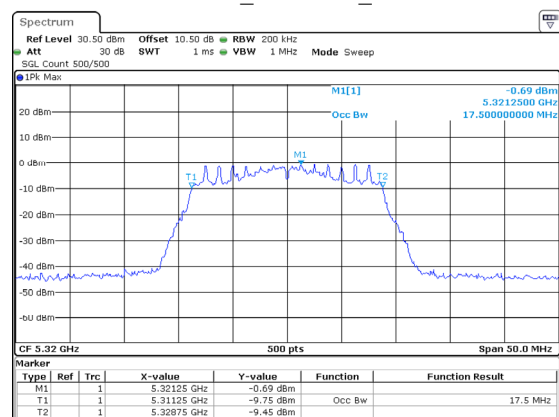
802.11ac20_5320MHz_Chain 2
