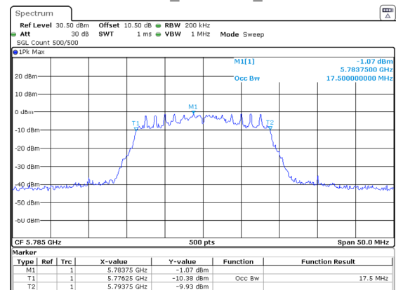
802.11ac20_5785MHz_Chain 1
