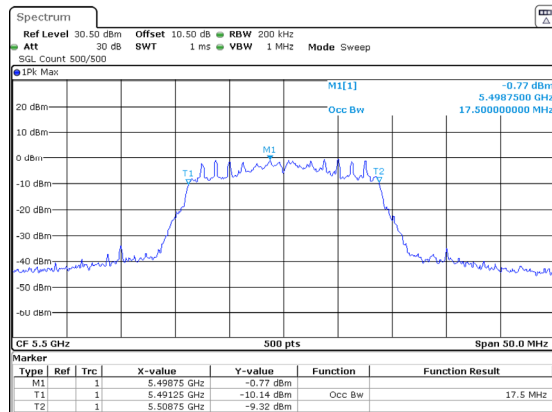
802.11ac20_5500MHz_Chain 1
