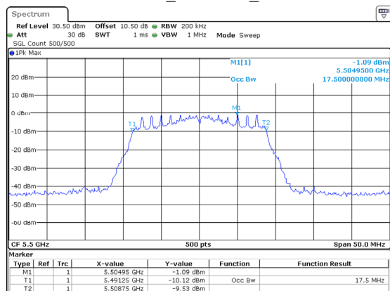
802.11ac20_5500MHz_Chain 2
