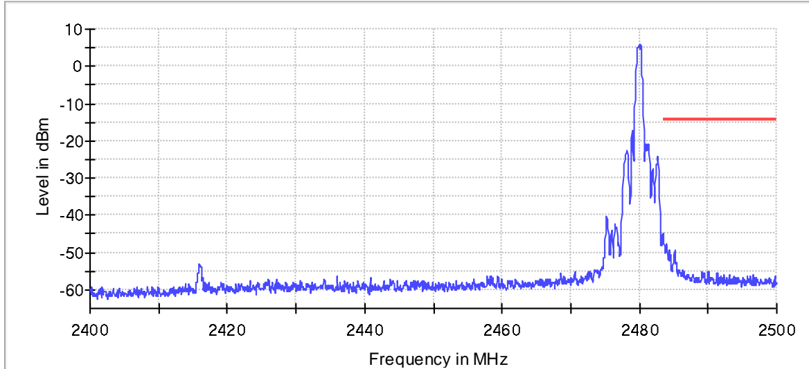
Band Edge
