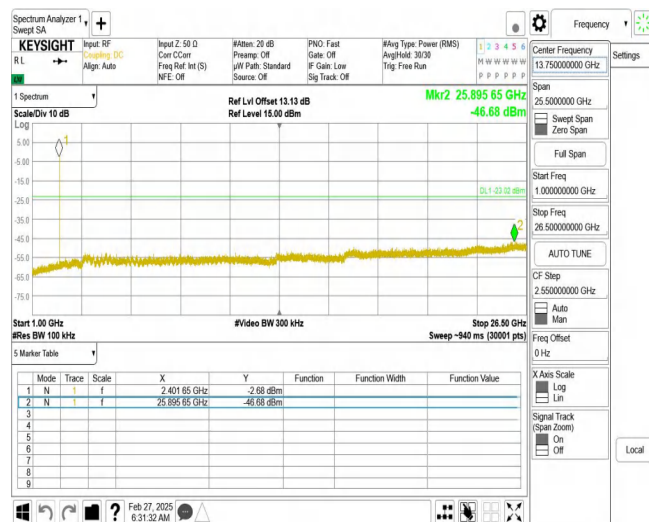
BLE_2M_Ant1_2402_1000~26500
