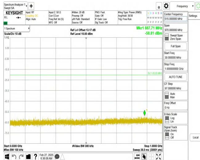
BLE_2M_Ant1_2480_30~1000
