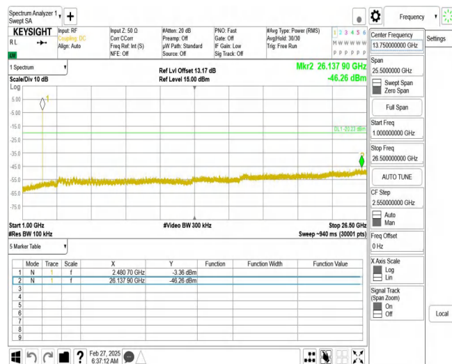
BLE_2M_Ant1_2480_1000~26500
