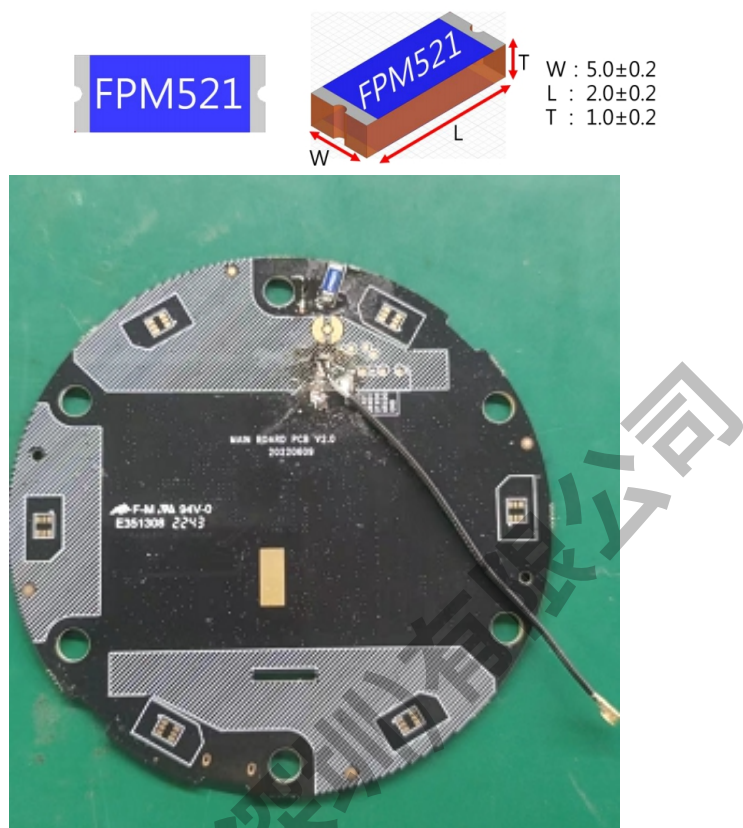
图 1 天线 Antenna
