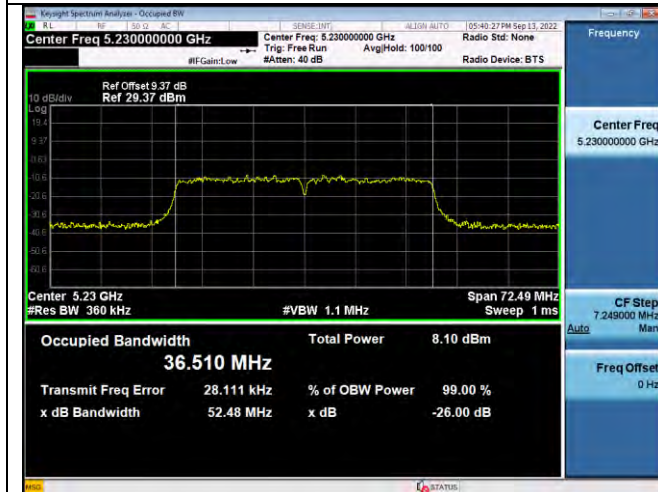
CH46-5230MHz
