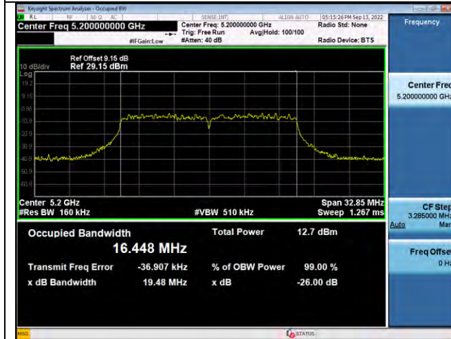
CH40-5200MHz
