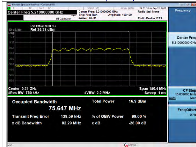
CH42 5210MHz
