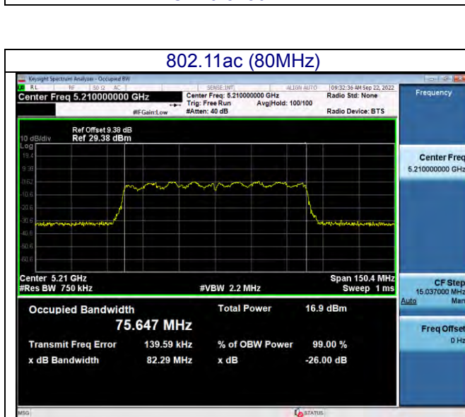
CH42 5210MHz
