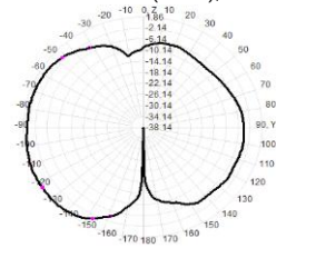
2420.0MHz Total(E2-YZ), Max= 1.36dB
