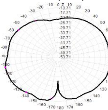
915.0MHz Total(E1-XZ), Max= -13.86dBi
