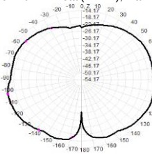
917.0MHz Total(E1-XZ), Max= -14.17dBi
