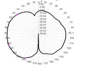
2430.0MHz Total(E2-YZ), Max= 0.61dB
