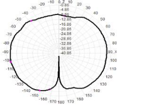
2490.0MHz Total(E1-XZ), Max= -4.19dBi
