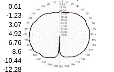
2430.0MHz Total(E1-XZ), Max= -2.68dB
