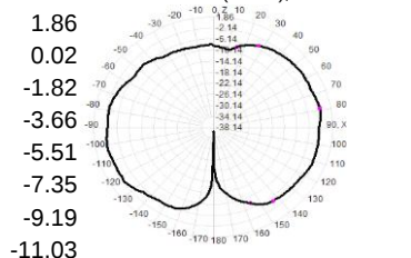
2420.0MHz Total(E1-XZ), Max= -2.10dB
