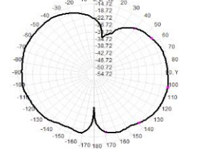
920.0MHz Total(E2-YZ), Max= -15.13dBi
