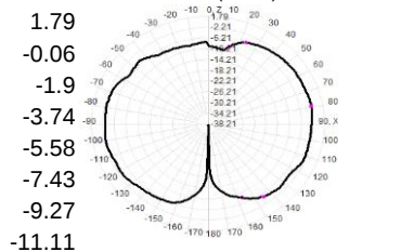
2410.0MHz Total(E1-XZ), Max= -1.99dB
