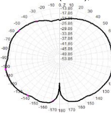
916.0MHz Total(E1-XZ), Max= -14.01dBi
