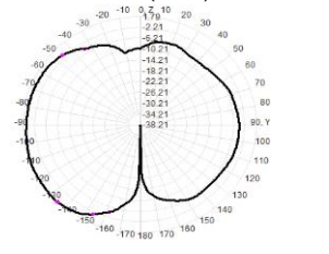
2410.0MHz Total(E2-YZ), Max= 1.86dB
