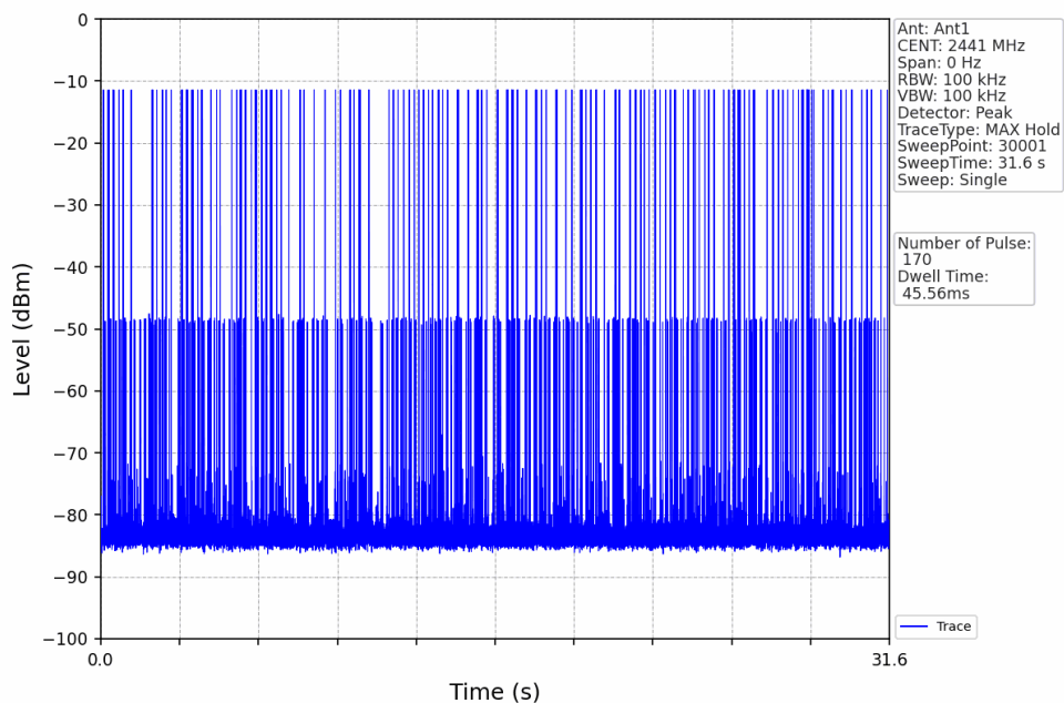
8DPSK_3DH3_HOPP_Ant1_NTNV
