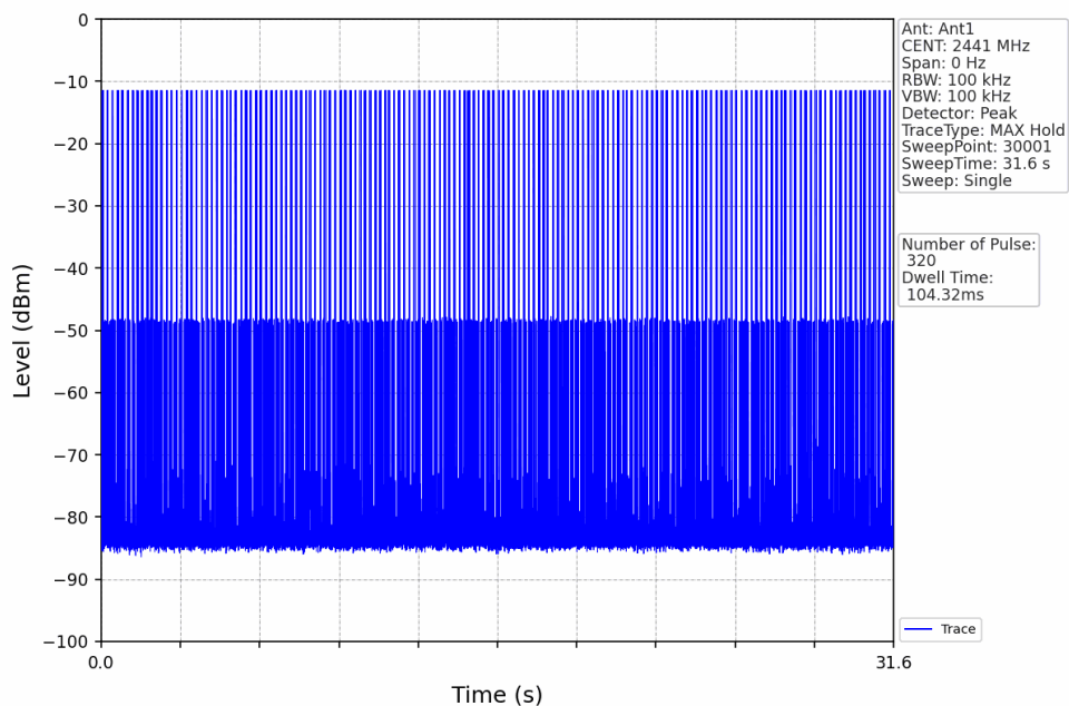
Pi/4DQPSK_2DH1_HOPP_Ant1_NTNV
