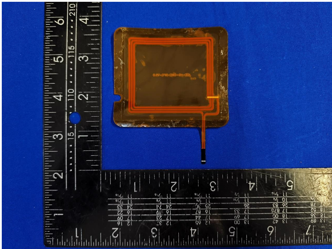
NFC antenna
