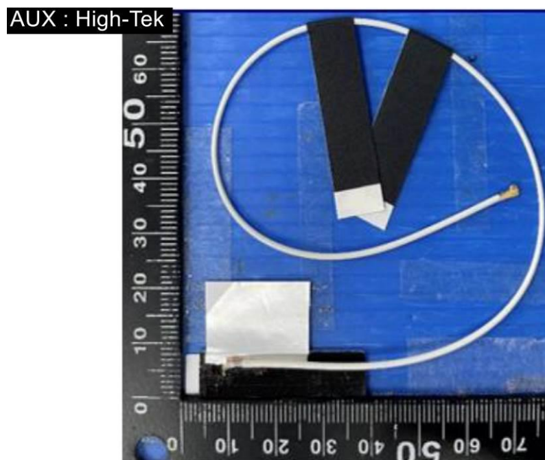
EUT Photo (14)
