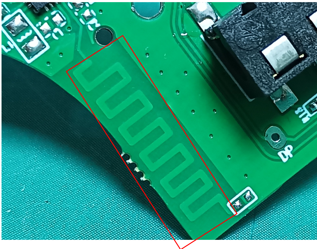
Antenna
