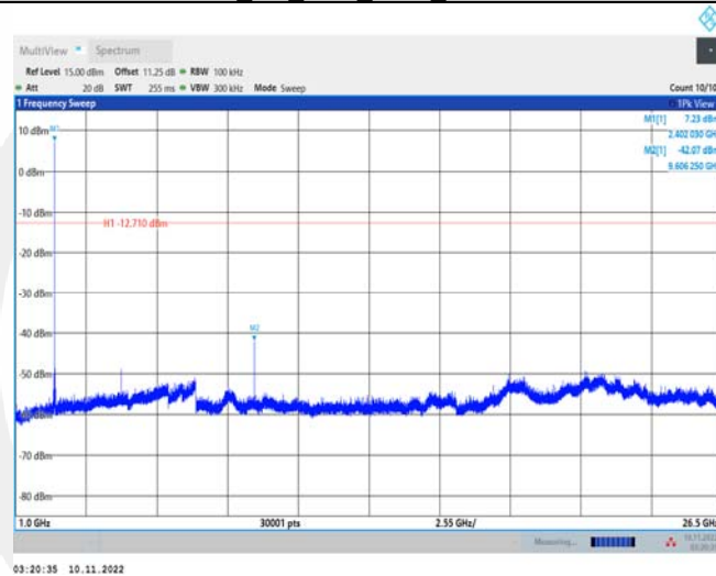
BLE_2M_Ant1_2402_1000~26500
