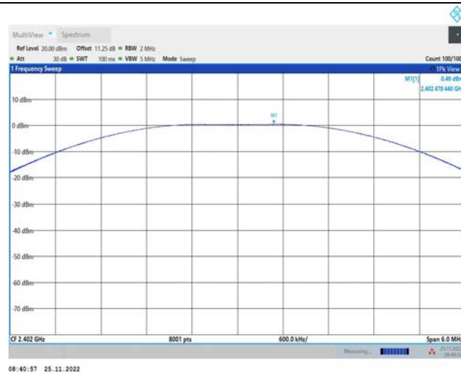
BLE_2M_Ant1_2402
