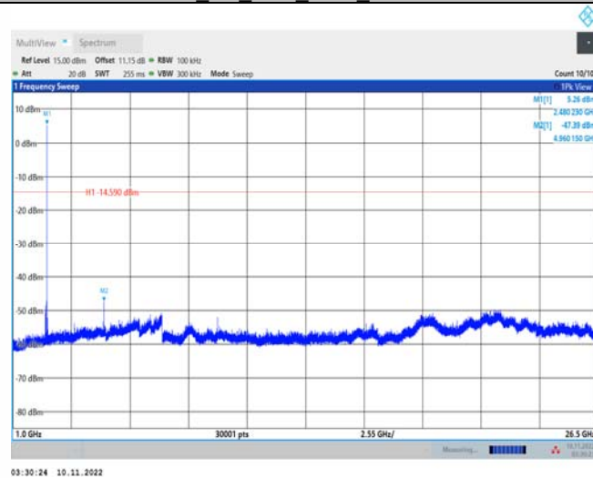
BLE_2M_Ant1_2480_1000~26500
