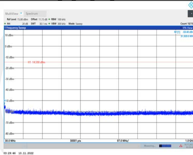
BLE_2M_Ant1_2480_30~1000
