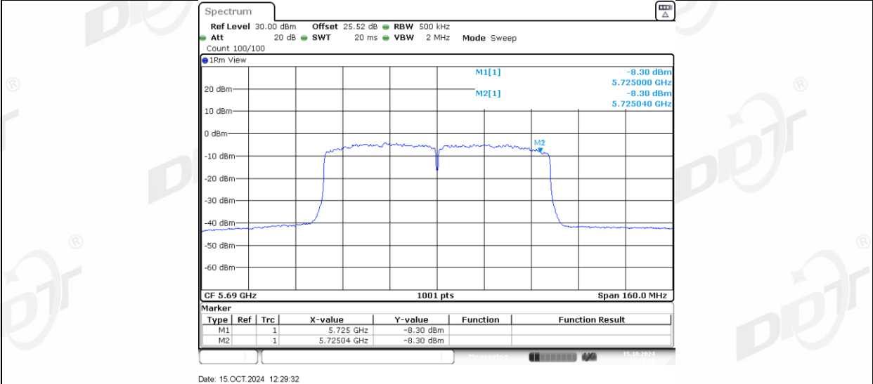
11AC80MIMO_Ant2_5690_UNII-3
