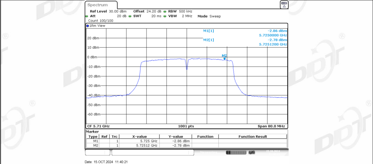
11N40MIMO_Ant2_5710_UNII-3
