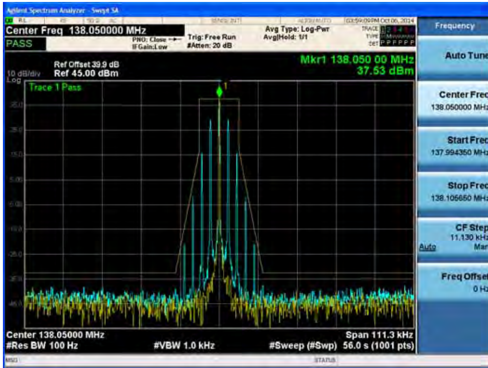
(11K0F3E _ 138.05 MHz)_High
