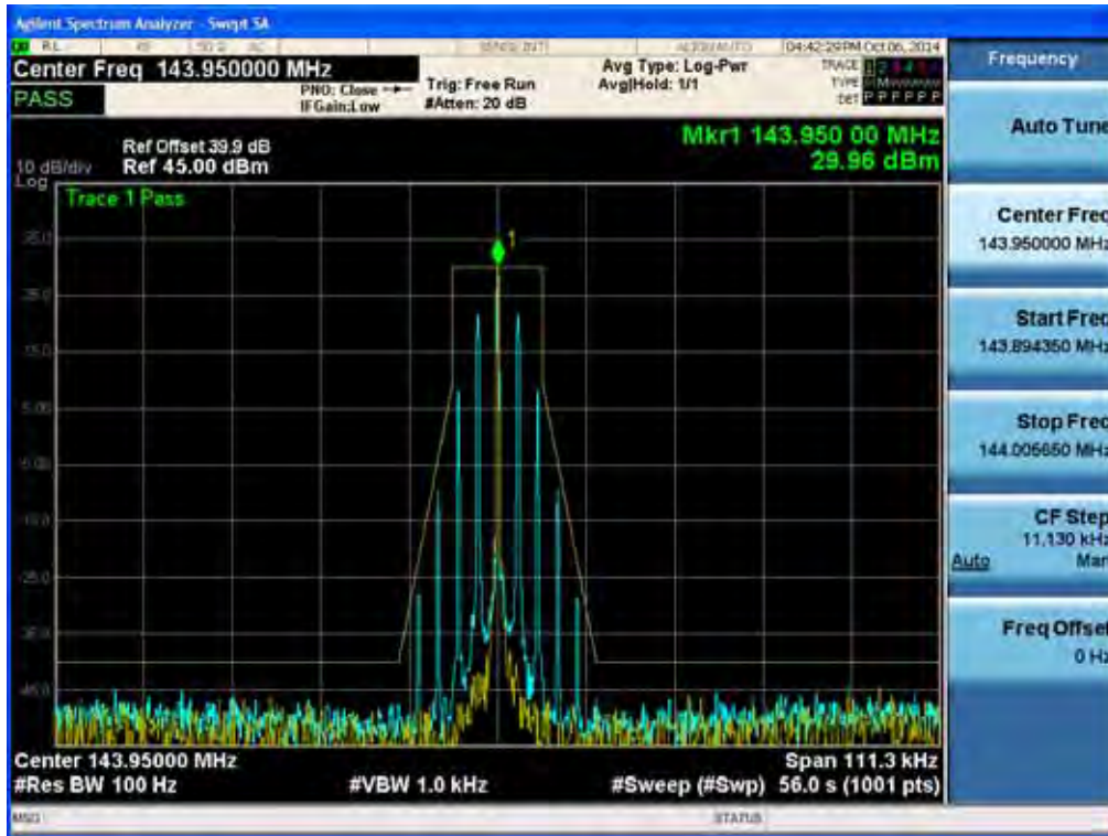
(11K0F3E _ 143.95 MHz)_Low
