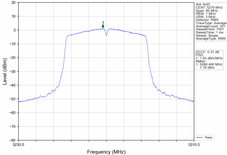
802.11n(HT40)_LCH_5270MHz_MIMO_NTNV
