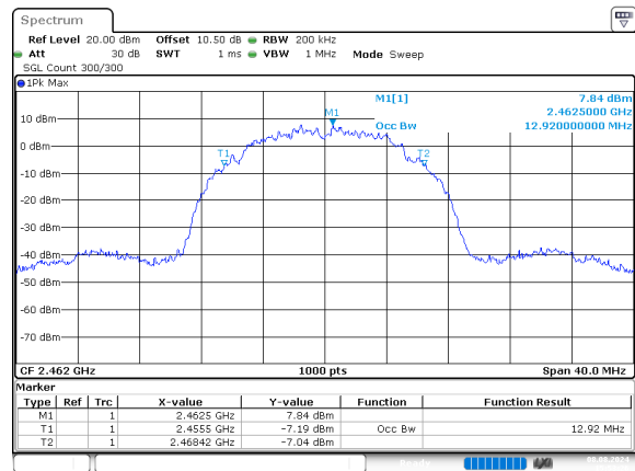
b_2462MHz
