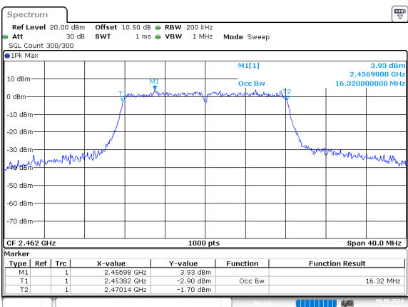
g_2462MHz
