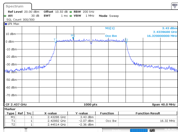
g_2437MHz
