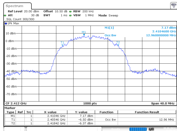
b_2412MHz
