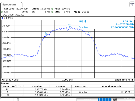
b_2437MHz
