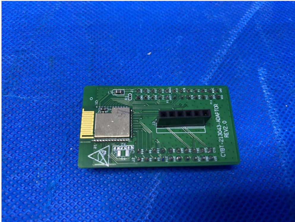
(3) EUT Photo (CYBT-213067-02)
