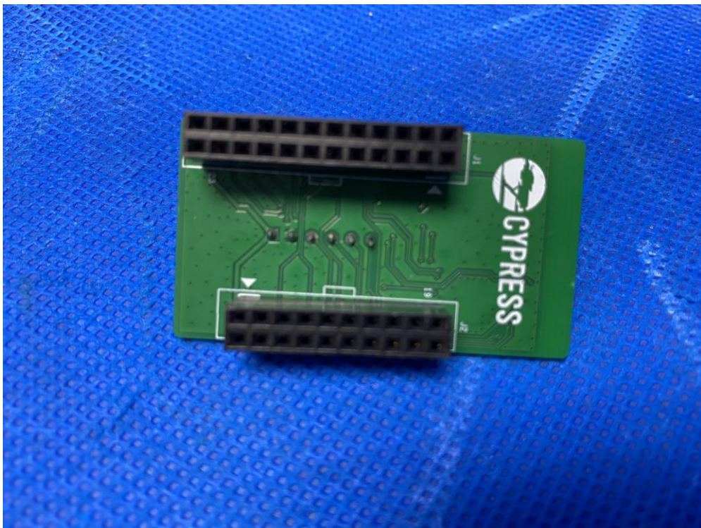
(2) EUT Photo (CYBT-213066-02)
