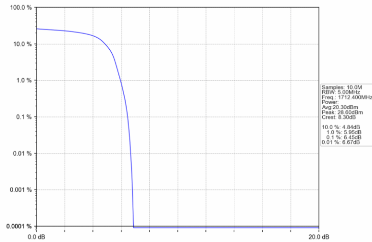
Band4 HSUPA LCH 1712.4MHz Subtest 1 NTNV
