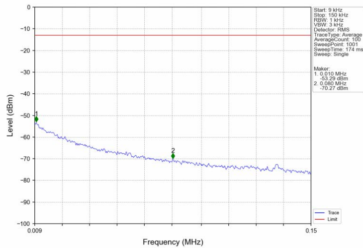
Band2 5MHz QPSK LCH 1852.5MHz RB 1 0 NTNv
