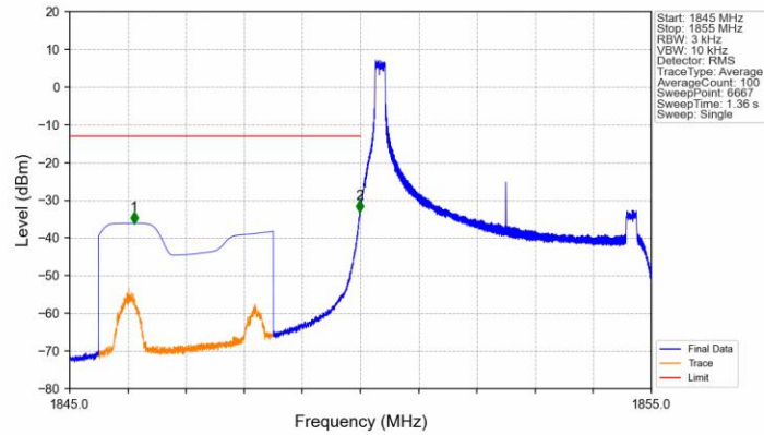
Band2 5MHz QPSK LCH 1852.5MHz RB 1 0 NTNv
