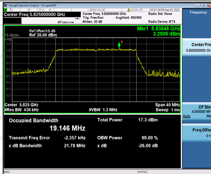
11AX20SISO_Ant2_5825
