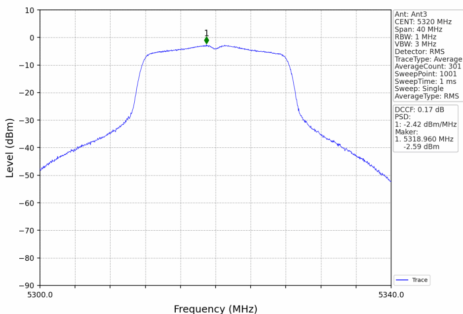
802.11a_HCH_5320MHz_Ant3_NTNV
