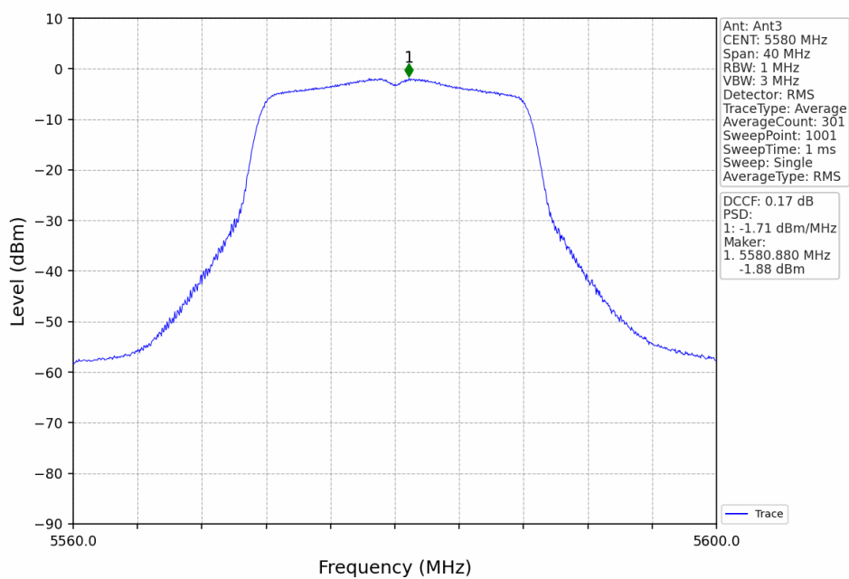
802.11a_MCH_5580MHz_Ant3_NTNV
