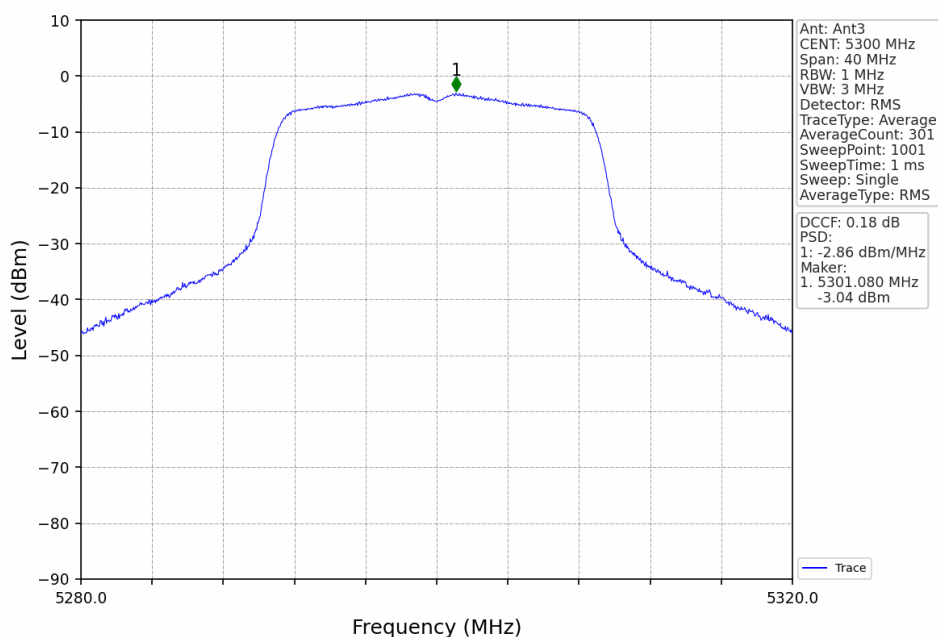
802.11n(HT20)_MCH_5300MHz_Ant3_NTNV
