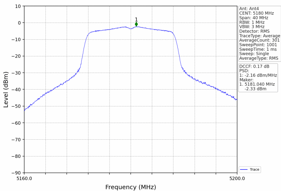
802.11a_LCH_5180MHz_Ant4_NTNV
