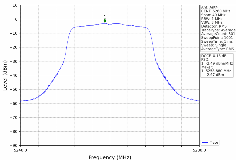
802.11n(HT20)_LCH_5260MHz_Ant4_NTNV
