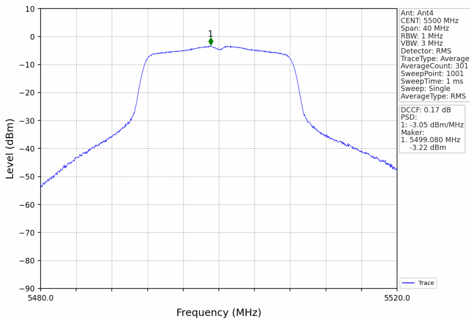
802.11a_LCH_5500MHz_Ant4_NTNV
