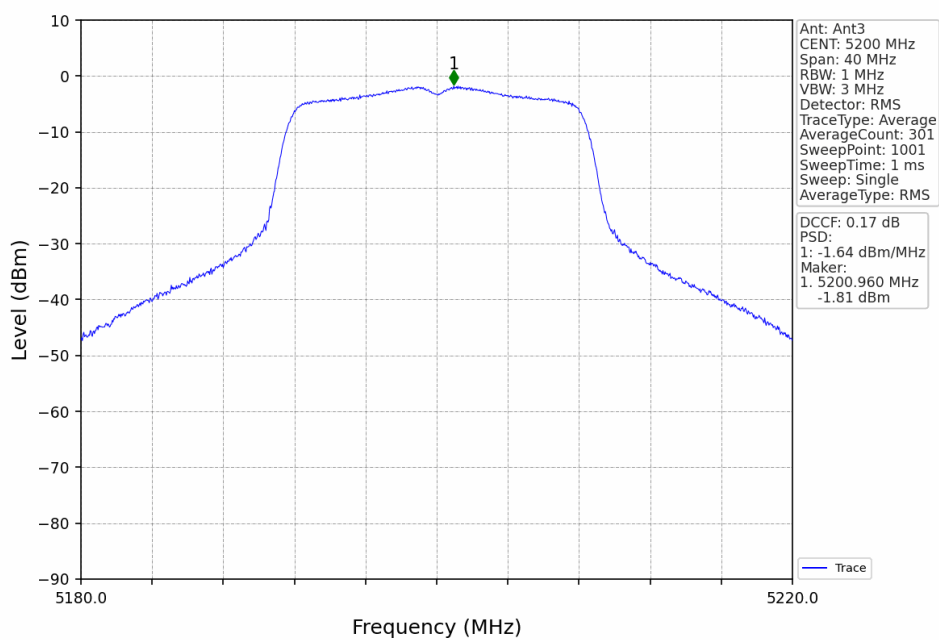
802.11a_MCH_5200MHz_Ant3_NTNV
