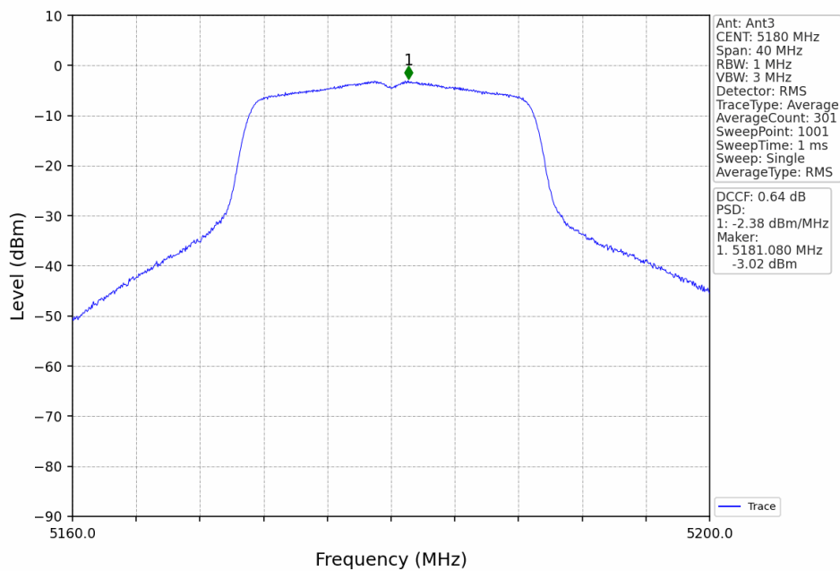
802.11n(HT20)_LCH_5180MHz_Ant3_NTNV
