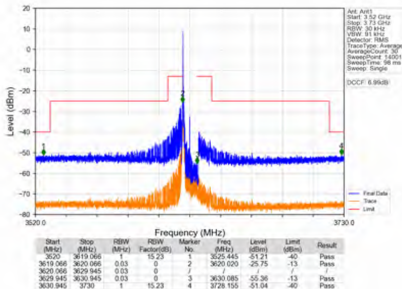
n78d 15kHz SISO NTNV 10MHz DFT-s-OFDM PI/2 BPSK 3625.005MHz Edge 1RB Left
