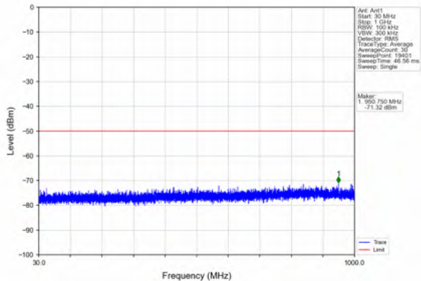
n78d_15kHz_SISO_NTNV_10MHz_CP-OFDM QPSK_3555MHz_Inner_1RB_Left
