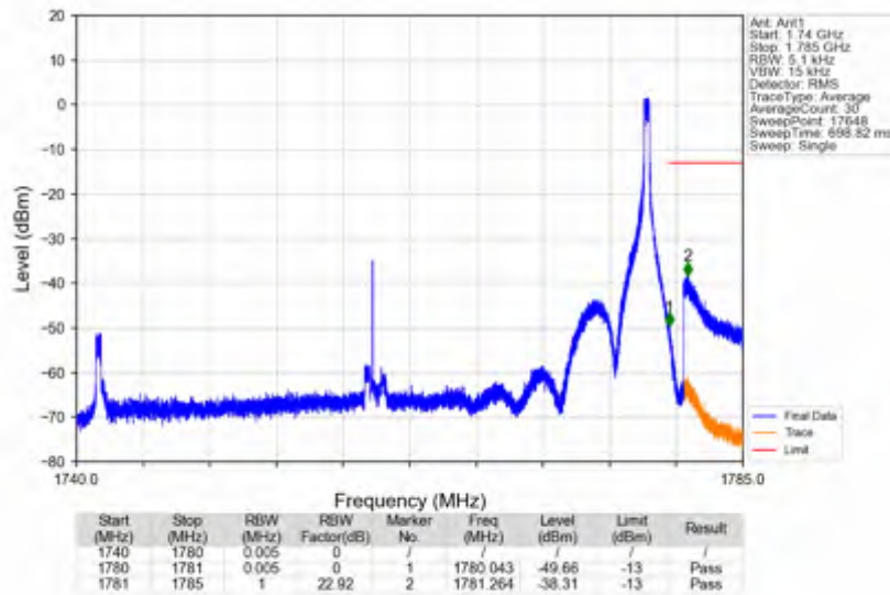
n66_30kHz_SISO_NTNV_40MHz_CP-OFDM QPSK_1760MHz_Inner_1RB_Right
