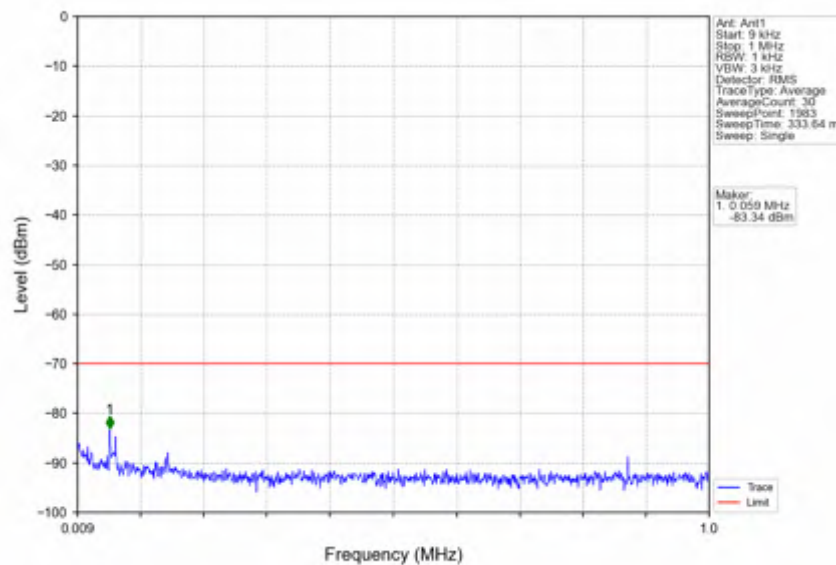
n78d_15kHz_SISO_NTNV_10MHz_DFT-s-OFDM PI/2 BPSK_3555MHz_Inner_1RB_Left
