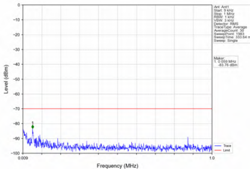
n78d_15kHz_SISO_NTV_10MHz_CP-OFDM_QPSK_3555MHz_Inner_1RB_Left
