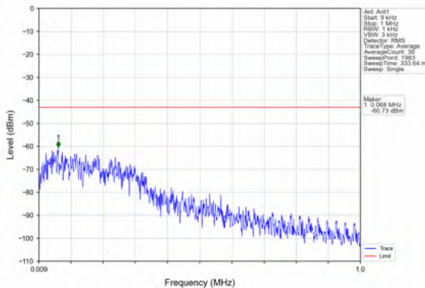
n66_30kHz_SISO_NTNV_40MHz_CP-OFDM QPSK_1760MHz_Inner_1RB_Right
