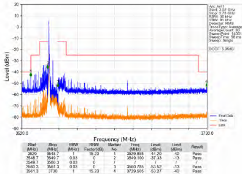
n78d_15kHz_SISO_NTV_10MHz_CP-OFDM_QPSK_3555MHz_Inner_1RB_Left
