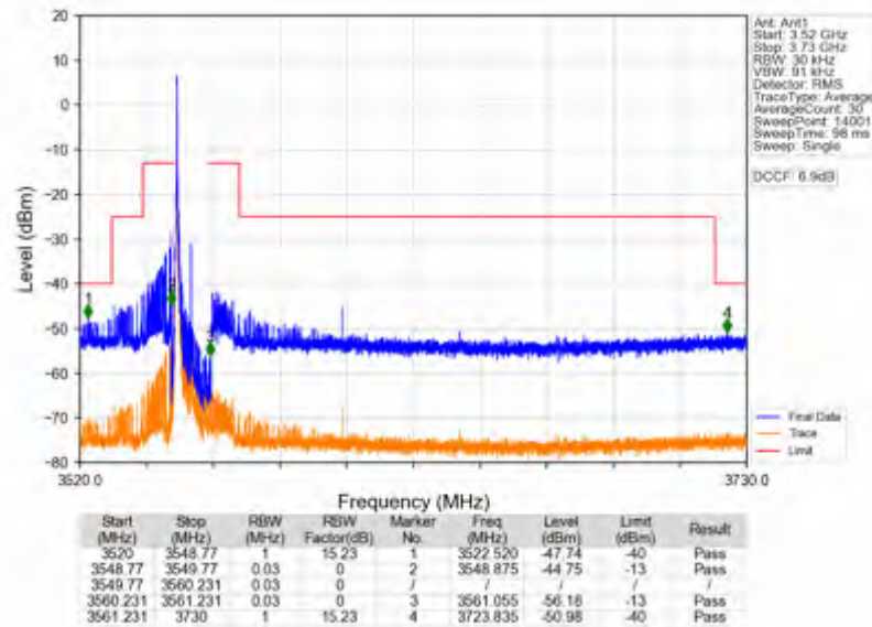
n78d_15kHz_SISO_NTNV_10MHz_DFT-s-OFDM PI/2 BPSK_3555MHz_Inner_1RB_Left
